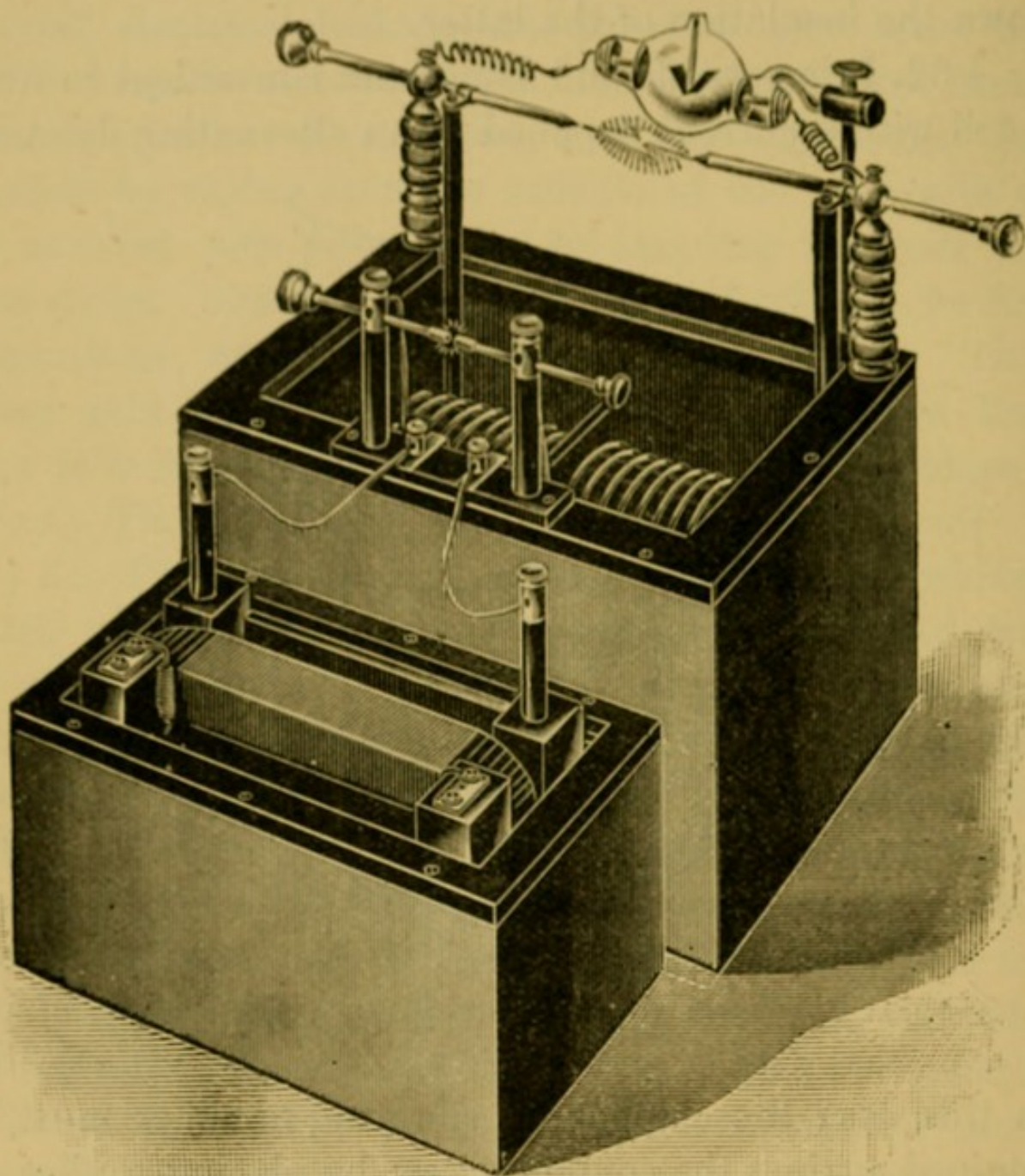
FIG. 20.-TESLA TRANSFORMER.
