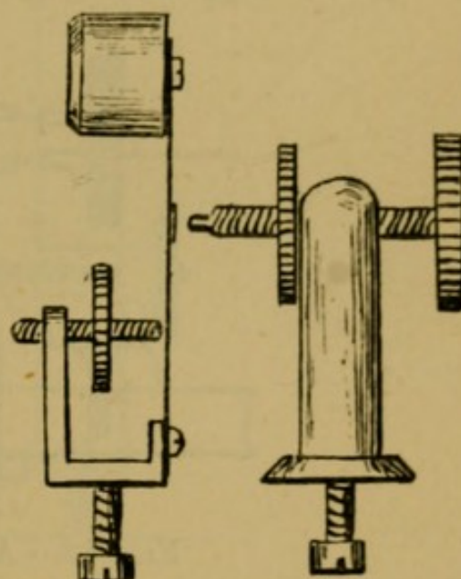
FIG. 11.—CONTACT-BREAKER.
