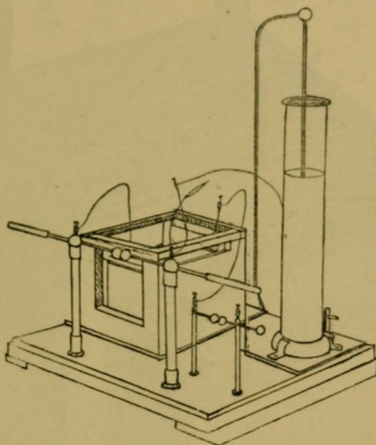
FIG. 19.—TESLA TRANSFORMER.
