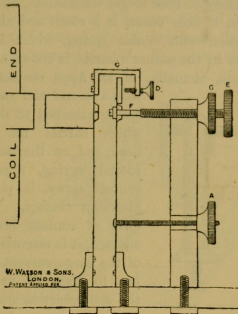
FIG. 13.—'VRIL' CONTACT-BREAKER.
