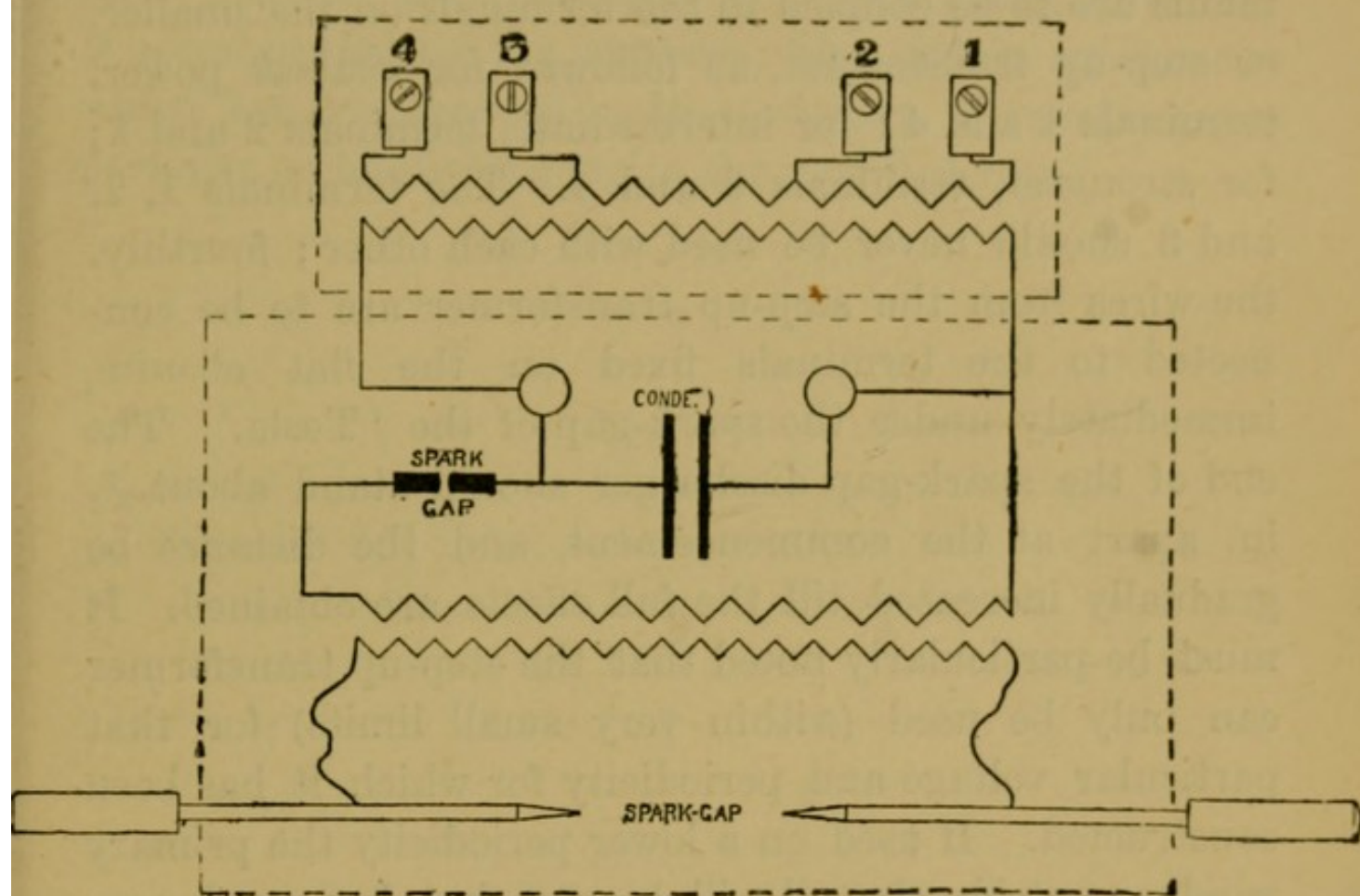
FIG. 21.—TESLA TRANSFORMER.
