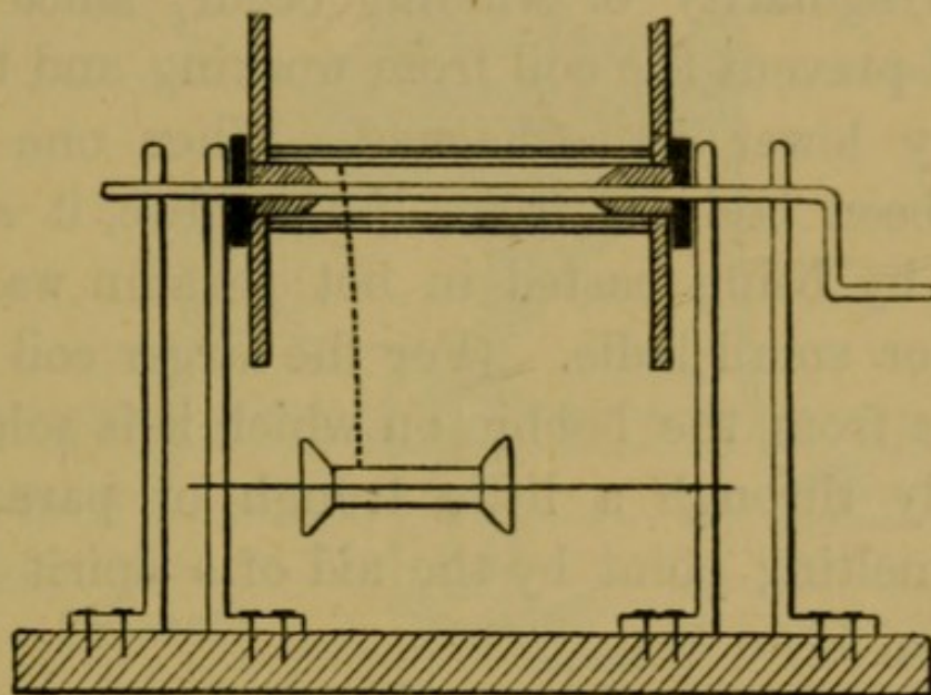
FIG. 4.—SIMPLE WINDER.
