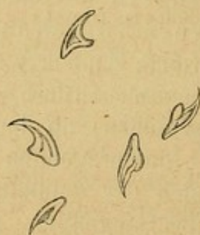
Fig. 11. Echinococcus-Häkchen.
