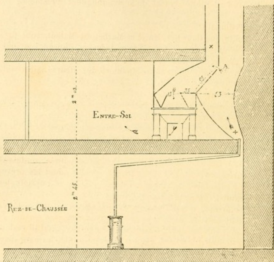
Fig. 4. — Plan du rez-de-chaussée et du premier étage.
