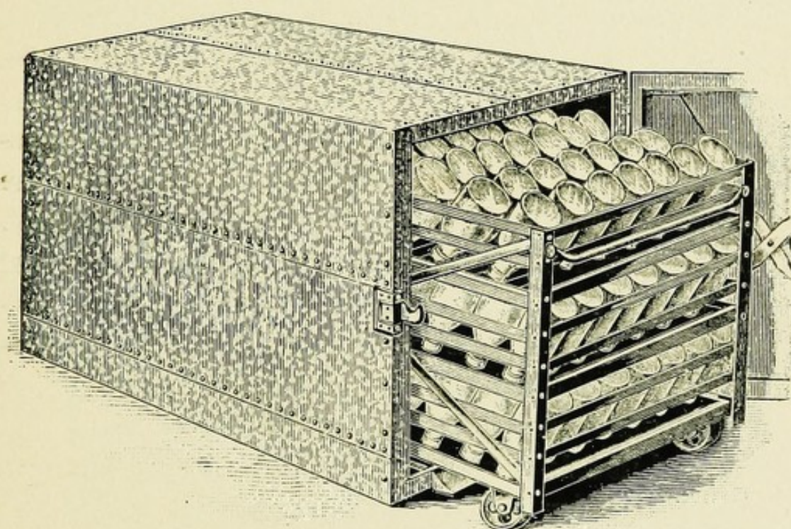
FIG. 26.—Bottle Sterilizer.
