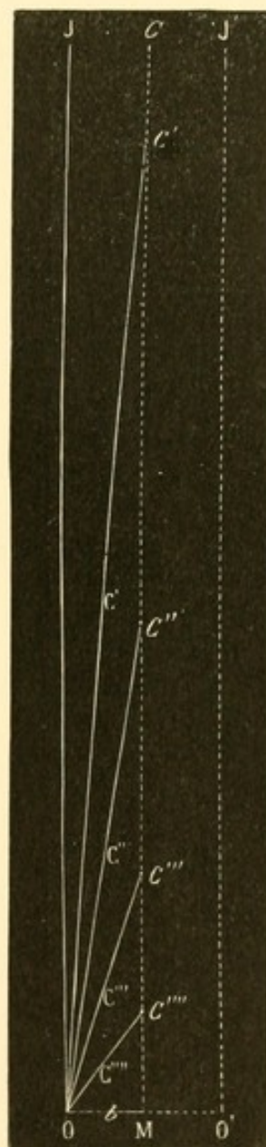
Metre angles of convergence (Landolt.)
