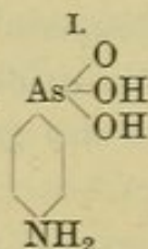
Paramidophenylarsinsäure.
