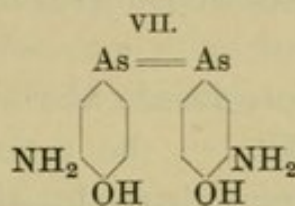
Dioxydiamidoarsenobenzol = 606.
