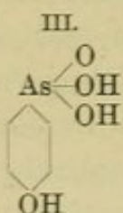
Paraoxyphenylarsinsäure
