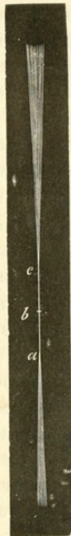
FIG. 53. — Ligne d'accommodation et point d'accommodation.
