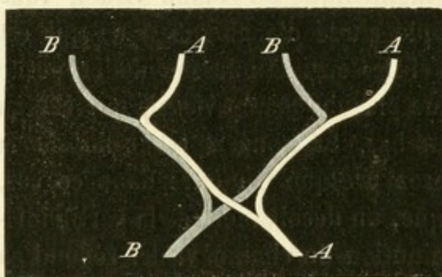
FIG. 33. — Distribution des nerfs optiques. Application à l'hémipie.
