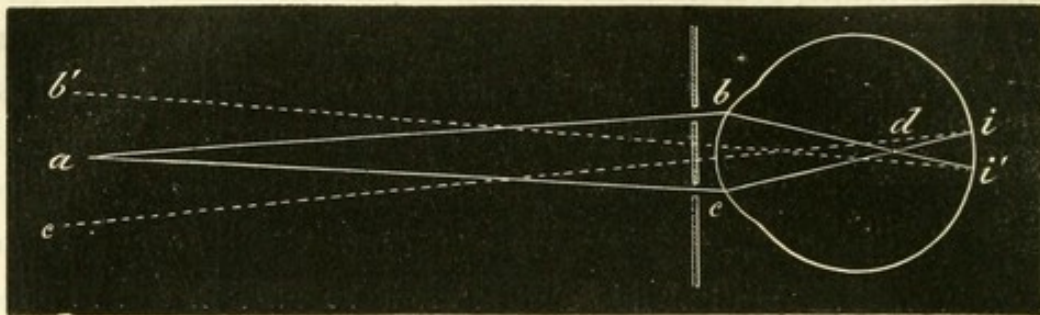
FIG. 51. — Expérience de Scheiner.
