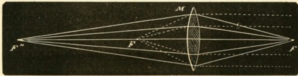
FIG. 41. — Foyers conjugués.
