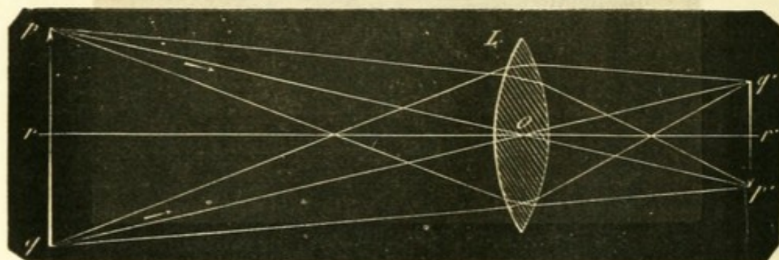
FIG. 44. — Construction d'une image dans une lentille.
