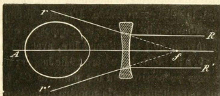
FIG. 62. — Mesure du degré de myopie.
