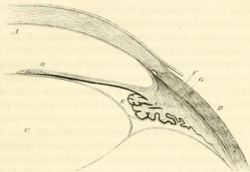
FIG. 60. — Coupe de l'œil destinée à montrer le muscle ciliaire. — A, cornée ; D, sclérotique ; H, canal de Schlemm ; G, portion radiée du muscle ciliaire ; F, portion circulaire du même muscle ; E, procès ciliaires ; C, cristallin ; B, iris.
