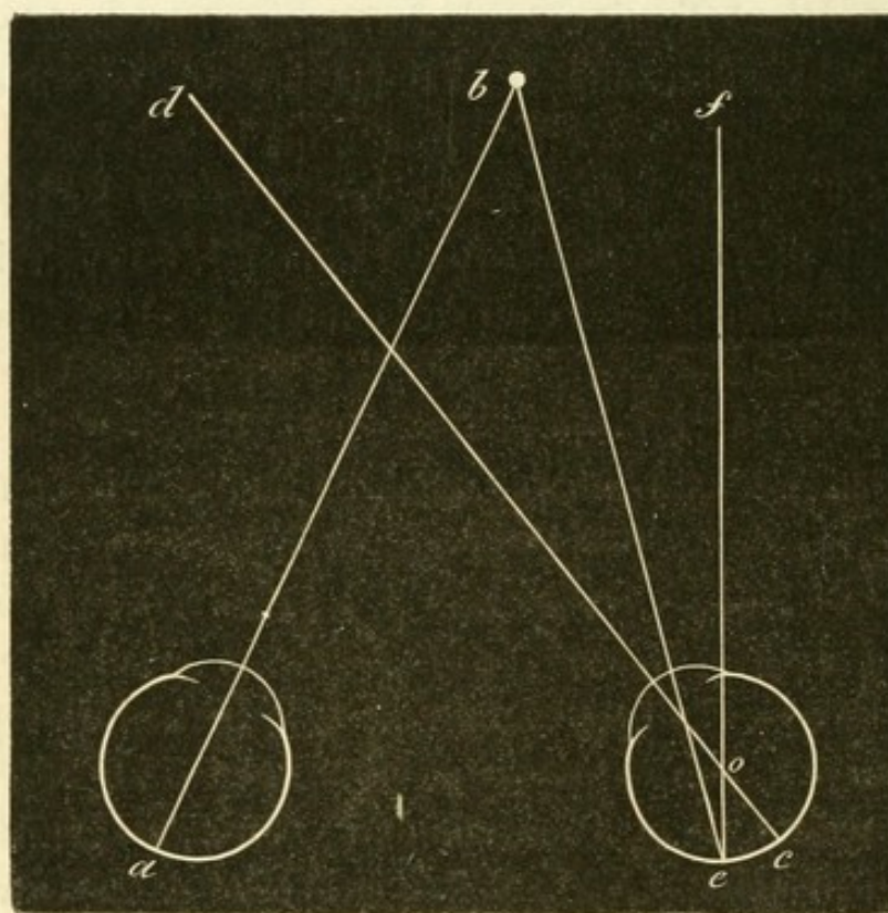
FIG. 67. — Strabisme convergent de l'œil droit. — Diplopie directe.
