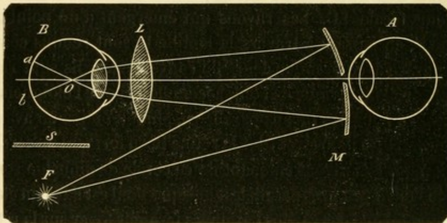
FIG. 13. — Éclairage par les miroirs concaves.
