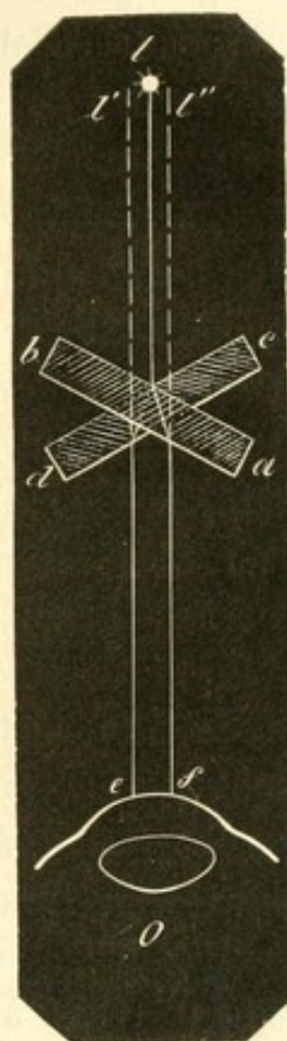
FIG. 59. — Principe de l'appareil de Helmholtz.
