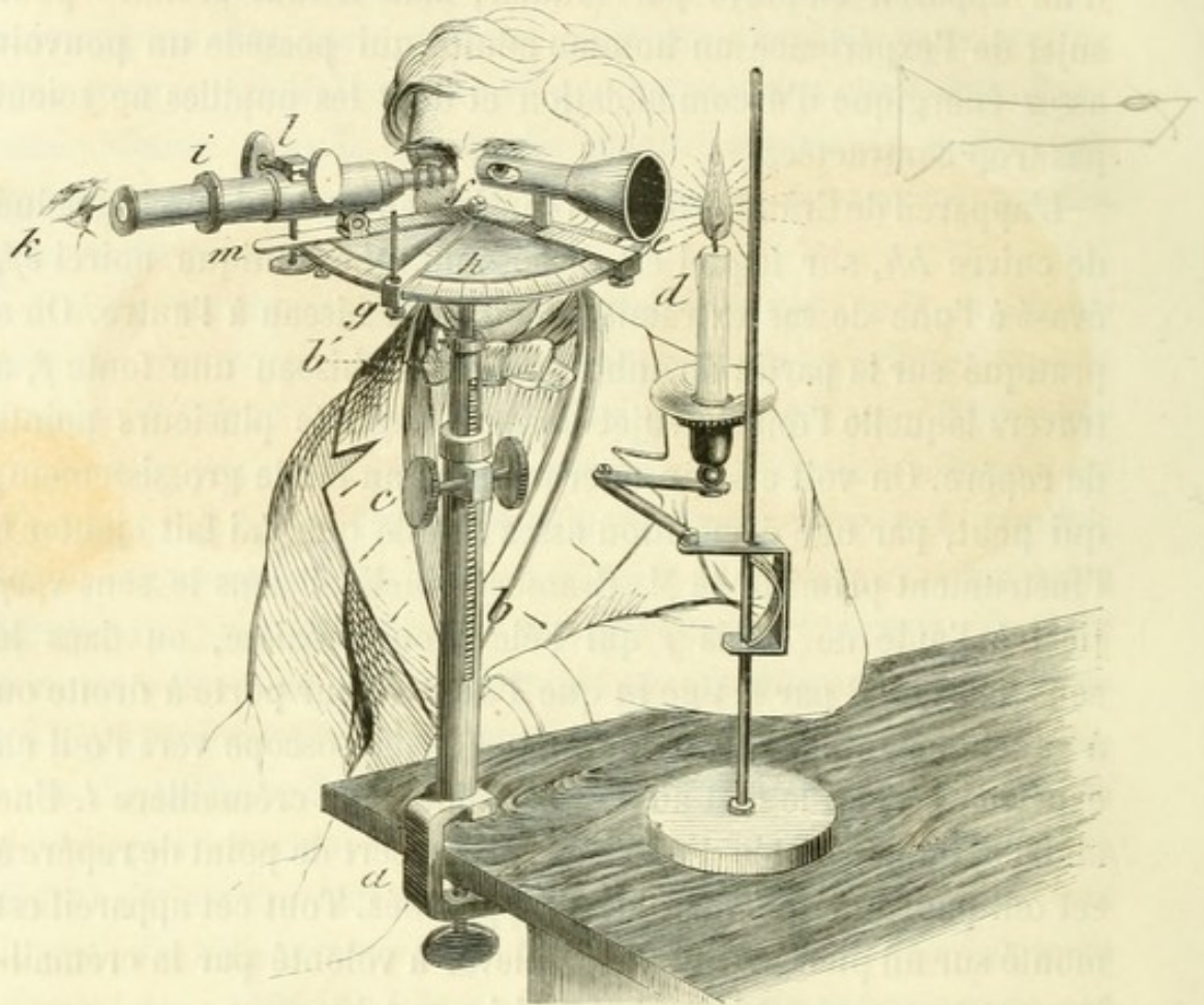
FIG. 54. — Appareil de Cramer pour démontrer les phénomènes intra-oculaires dans l'accommodation de l'œil.
