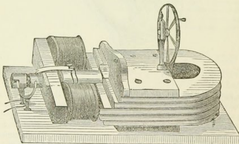
Saxton-Ettinghausen Apparatus.
