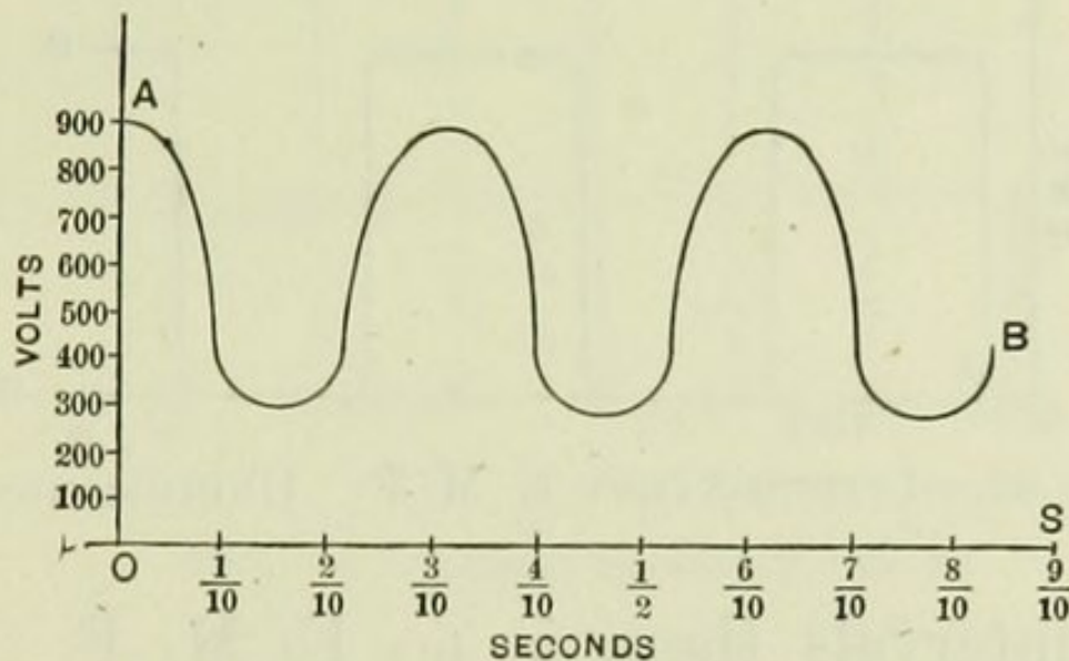
FIG. 41.—PULSATORY E. M. F.
