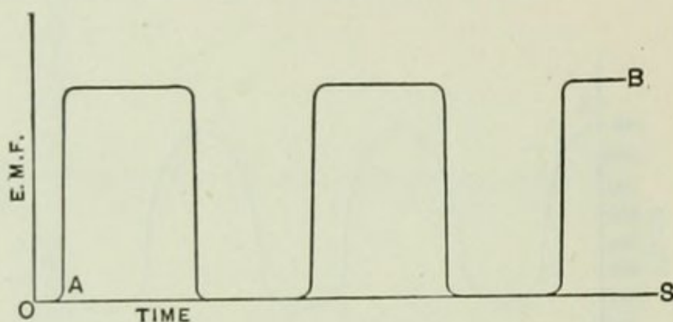
FIG. 42.—INTERMITTENT E. M. F. UNIDIRECTIONAL.
