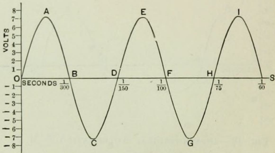
FIG. 49.—SINUSOIDAL E. M. F.
