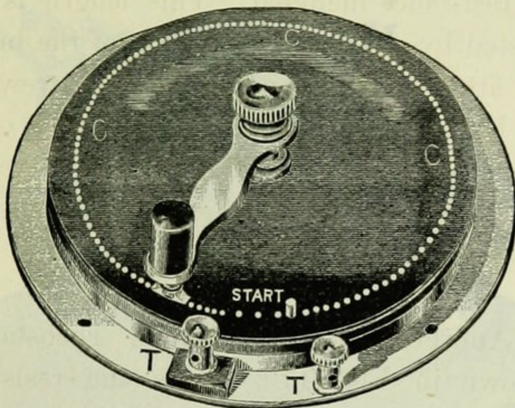
FIG. 119.—CARBON RHEOSTAT.
