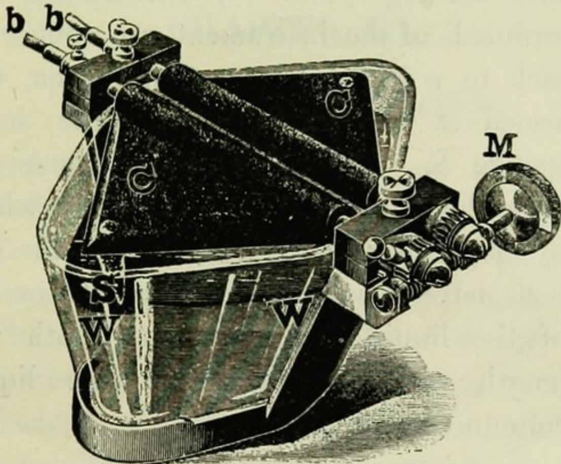
FIG. 121.—WATER RHEOSTAT.
