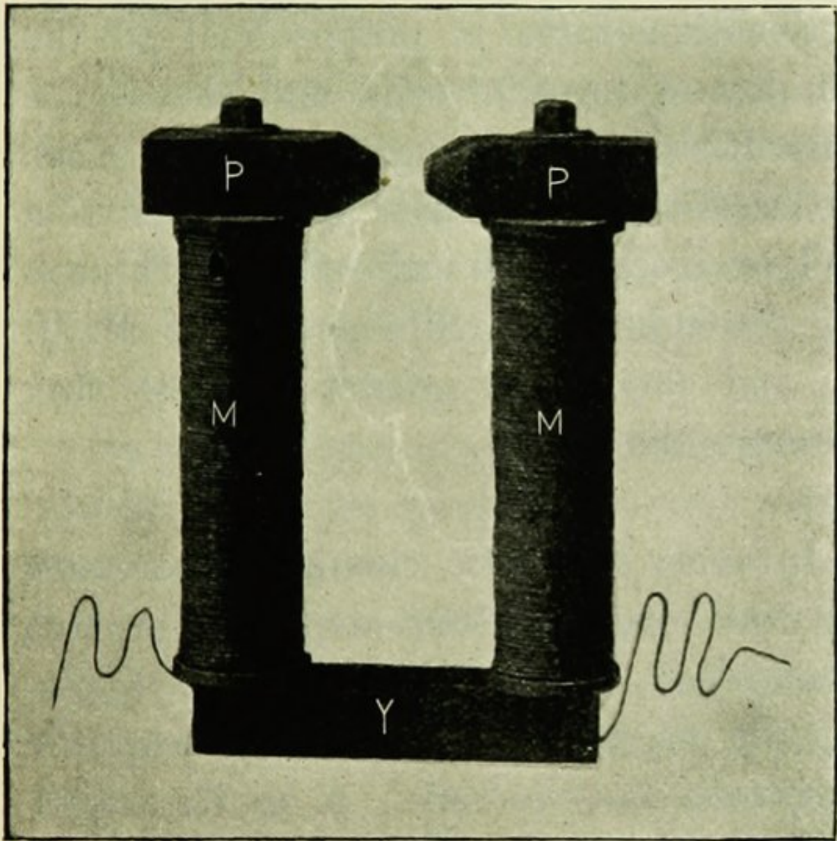
FIG. 81.—ELECTROMAGNET.
