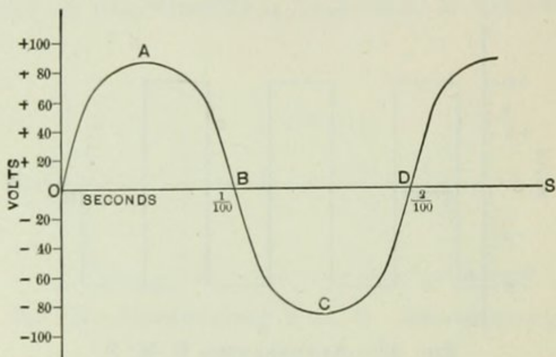
FIG. 44.—SYMMETRICAL ALTERNATING E. M. F.
