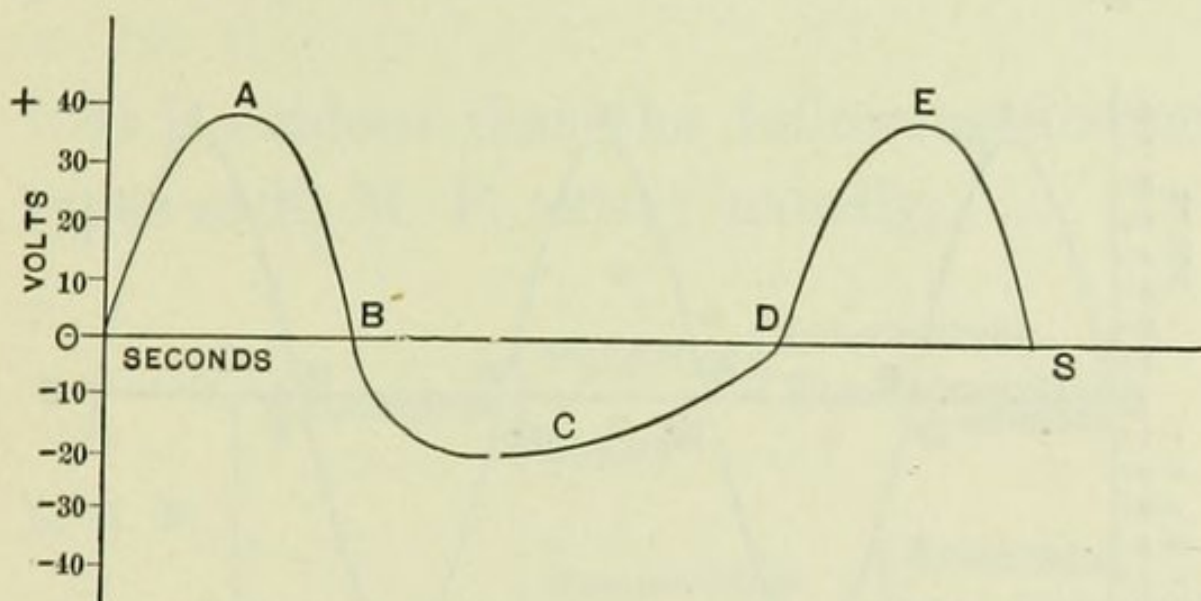
FIG. 48.—DISSYMMETRICAL ALTERNATING E. M. F.
