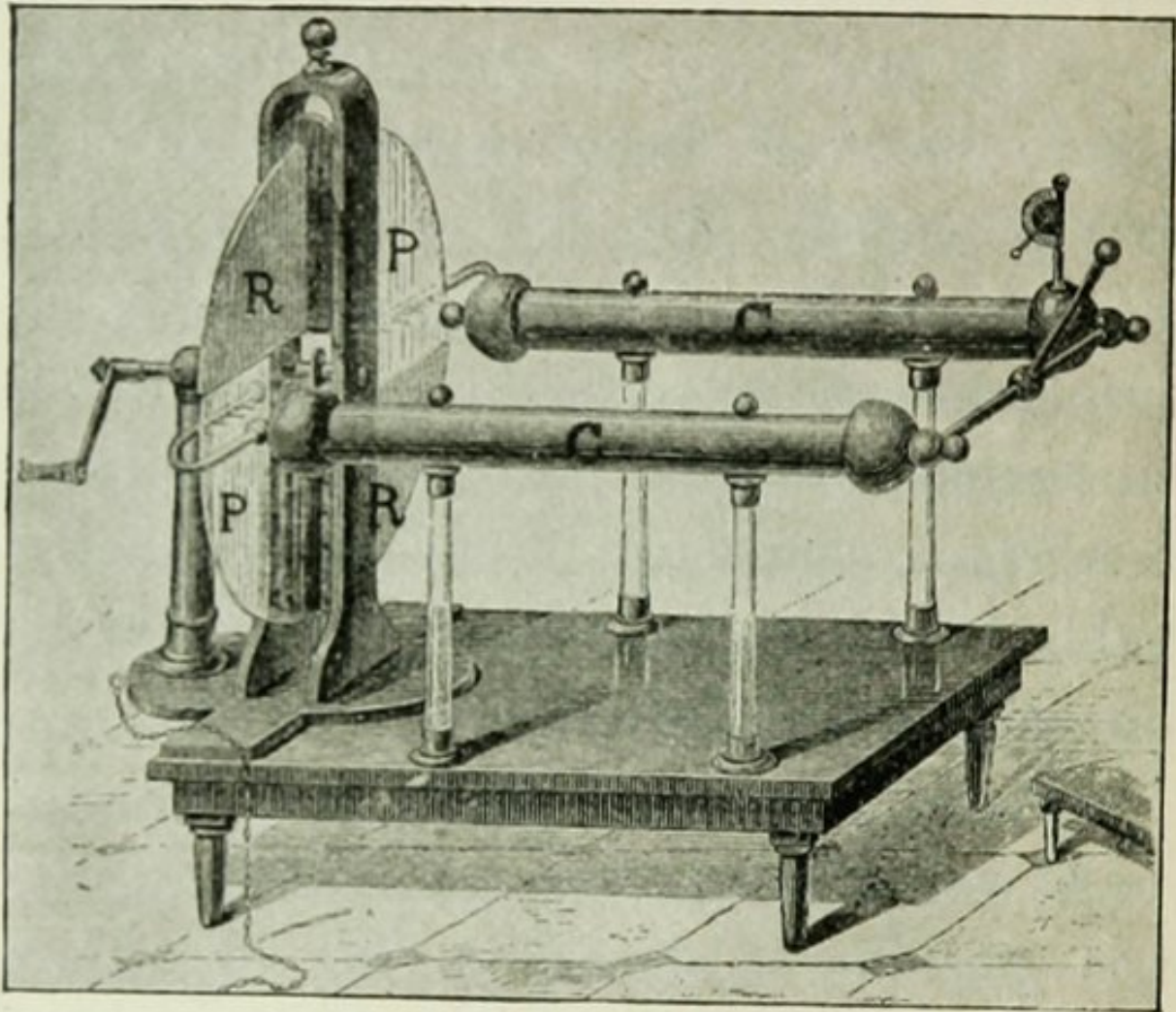
FIG. 52.
