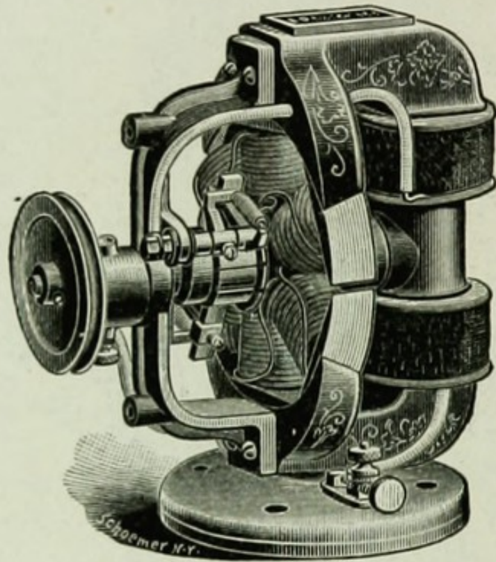
FIG. 110.—ELECTROMAGNETIC MOTOR.
