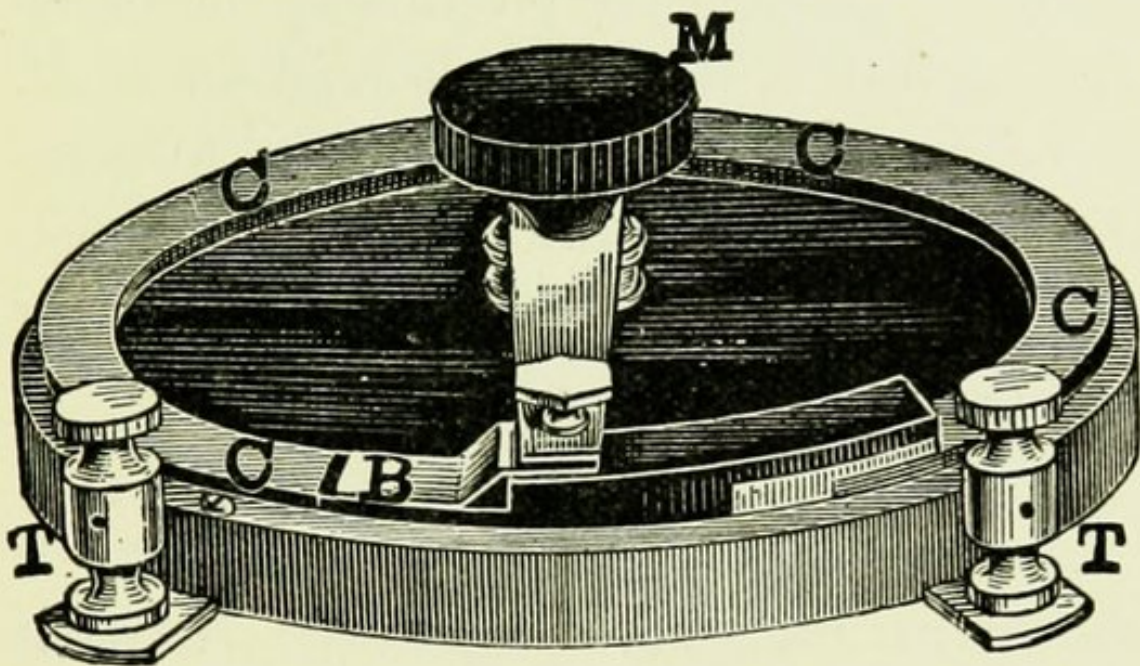
FIG. 118.—CARBON RHEOSTAT.
