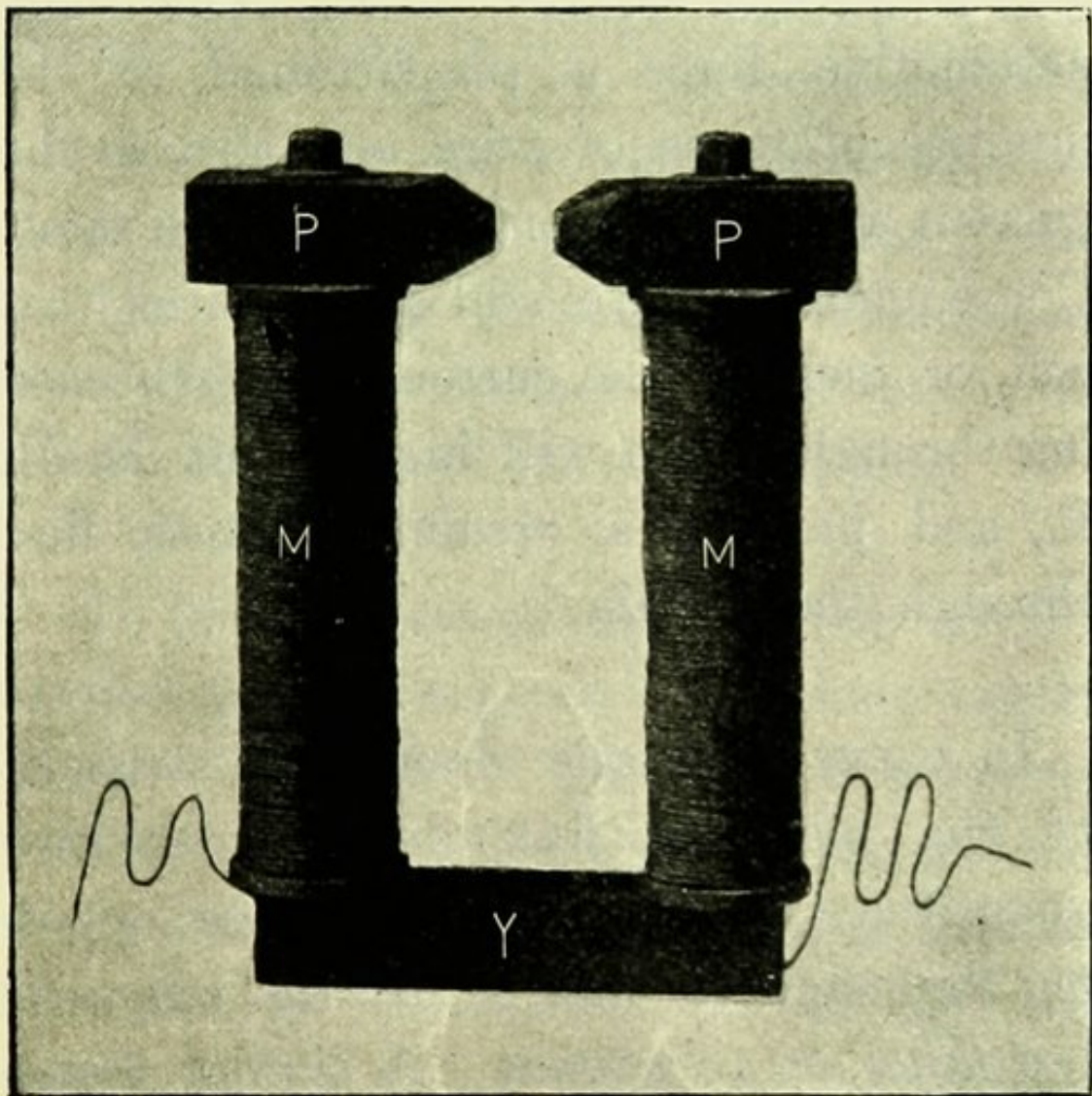
FIG. 81.—ELECTROMAGNET.
