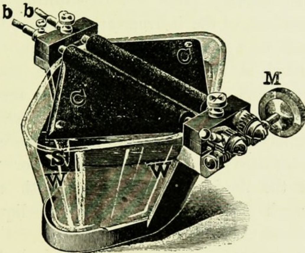
FIG. 121.—WATER RHEOSTAT.
