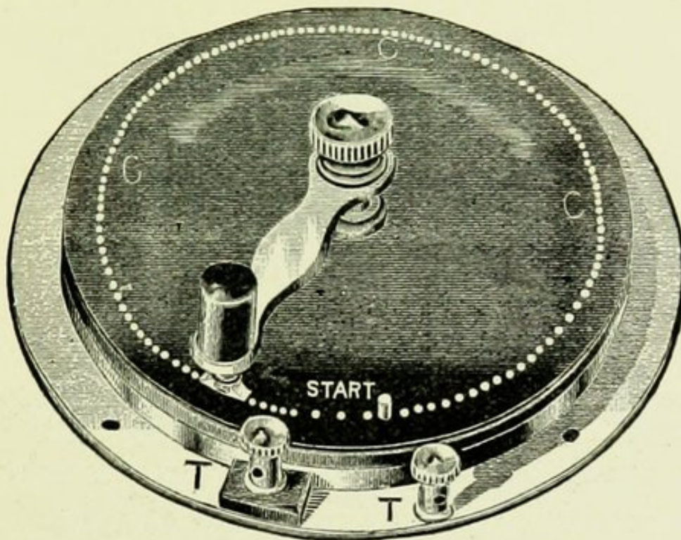
FIG. 119.—CARBON RHEOSTAT.
