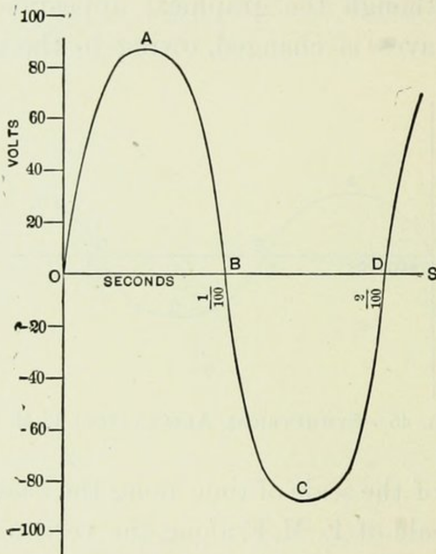
FIG. 46.—SYMMETRICAL ALTERNATING E. M. F.
