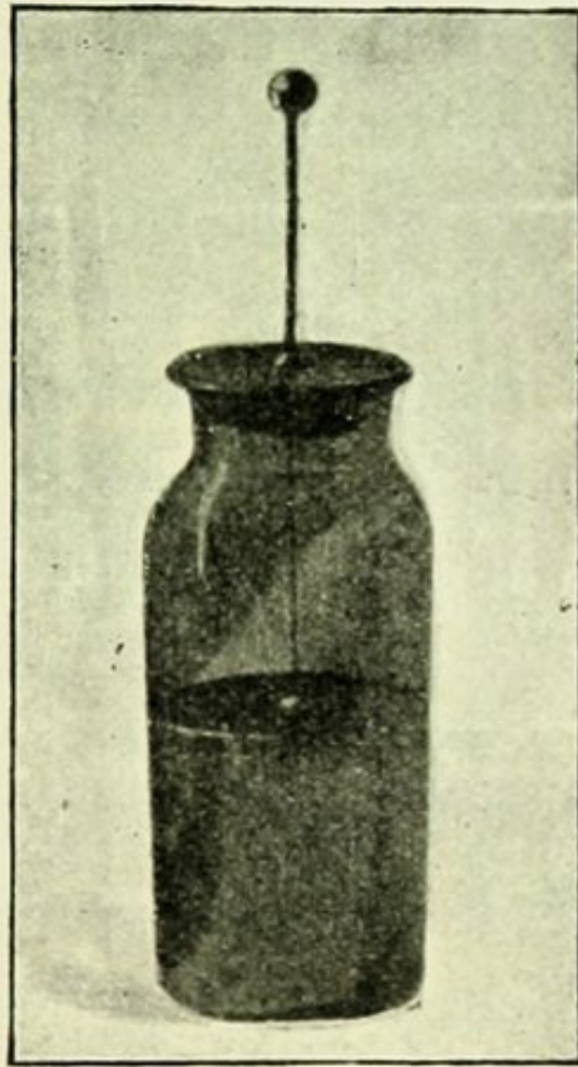
FIG. 70.—LEYDEN JAR.
