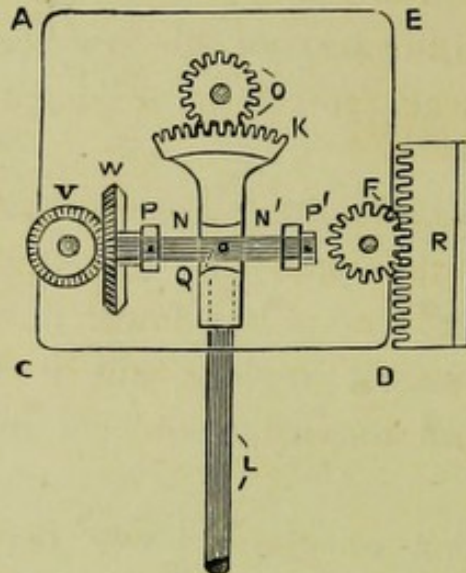
FIG. 3.—Sectional plan.
