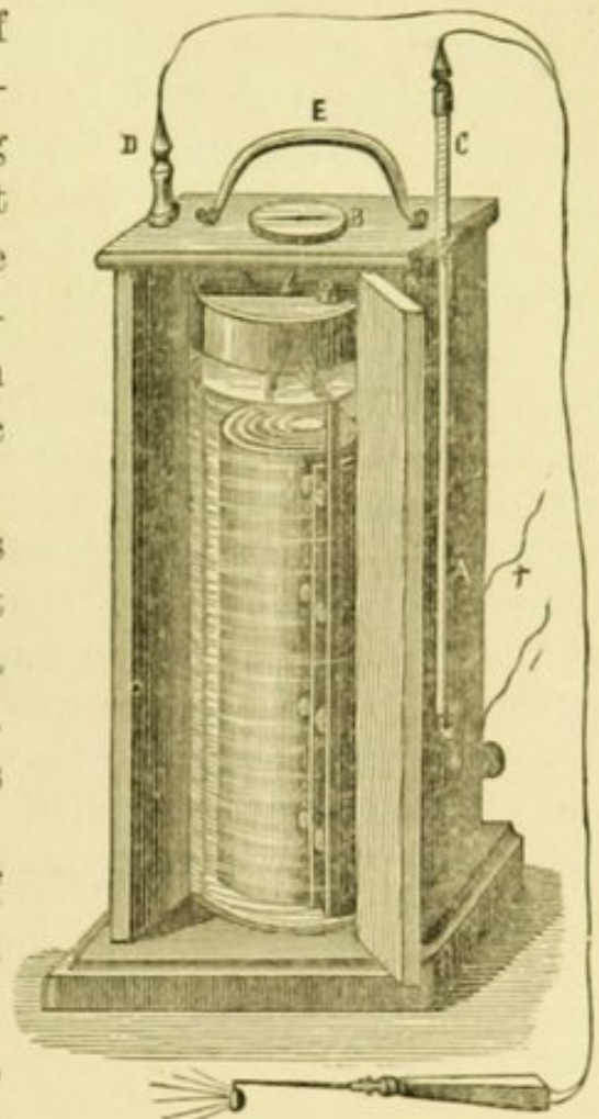
FIG. 28.—Trouve's Galvanic Accumulator.
