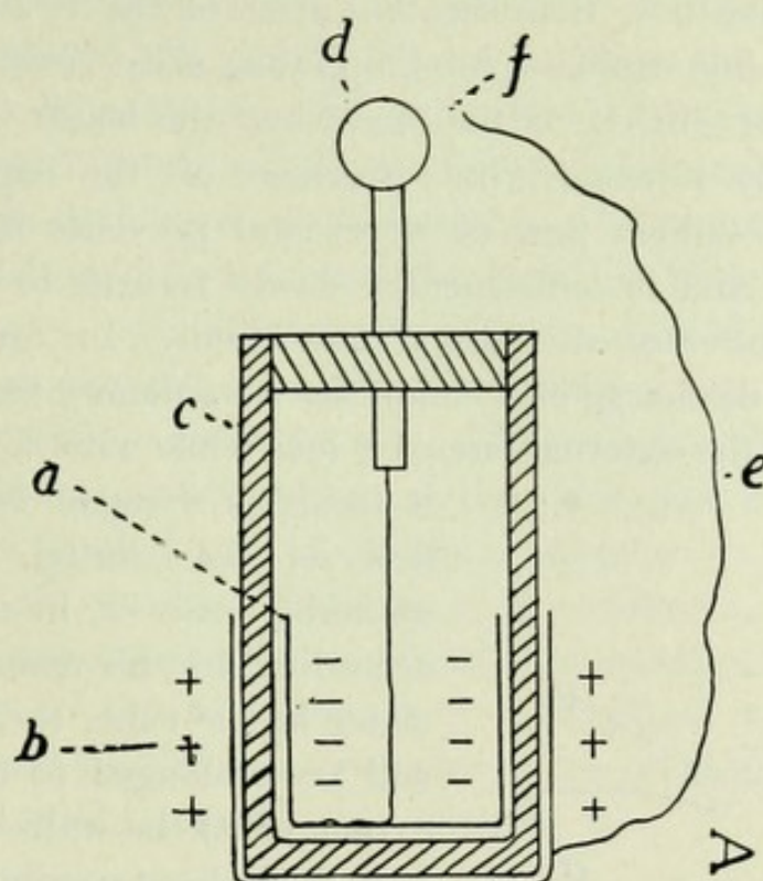
FIG. 23.—Leyden Jar, or Condenser.
