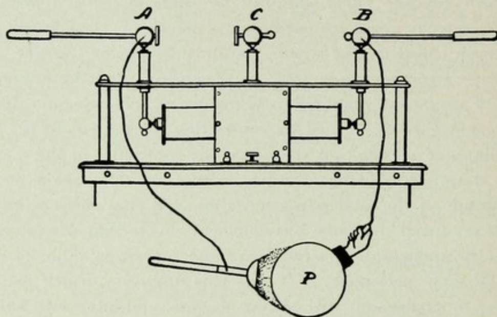
FIG. 117.—Tesla-Effluve.
