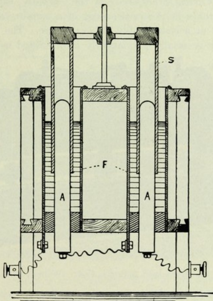
FIG. 32.—Nodon Valve, or Rectifier. (Williams.)
