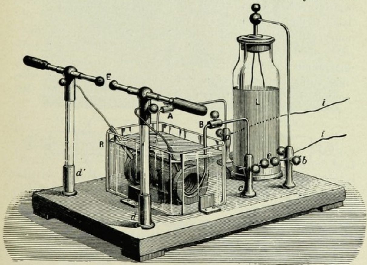
FIG. 4.—Miniature Tesla Apparatus. (E. Ducretet.)
