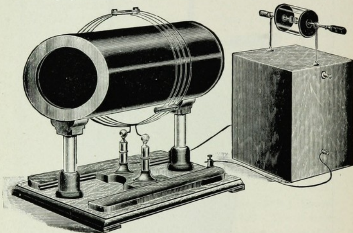
FIG. 45.—Gaiffe’s Bipolar Resonator.
