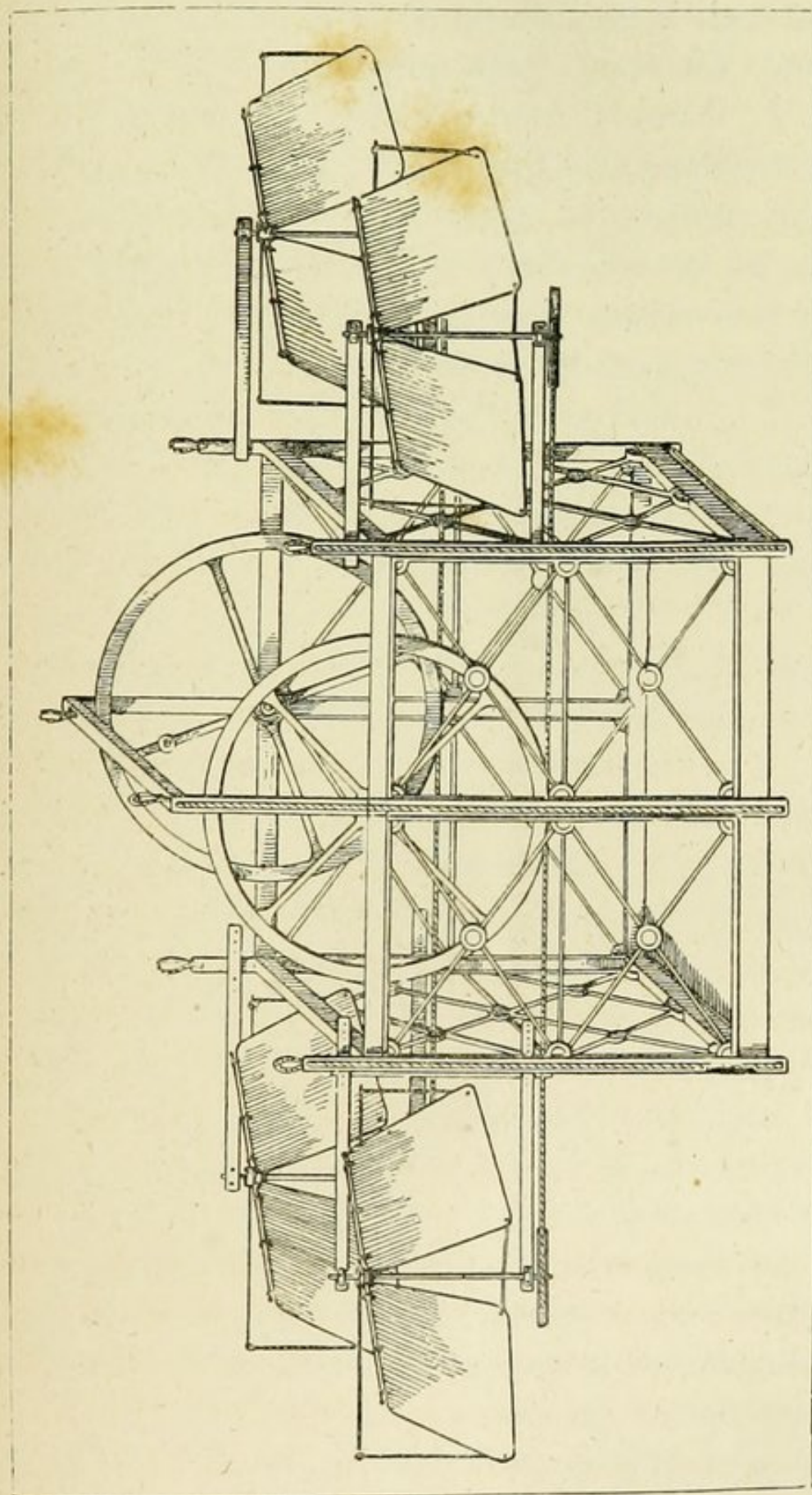
Fig. 63. — Nacelle de ballon à ailes tournantes du docteur Van Hecke, destinée à monter ou à descendre dans l'atmosphère sans perdre de gaz et sans jeter de lest.
