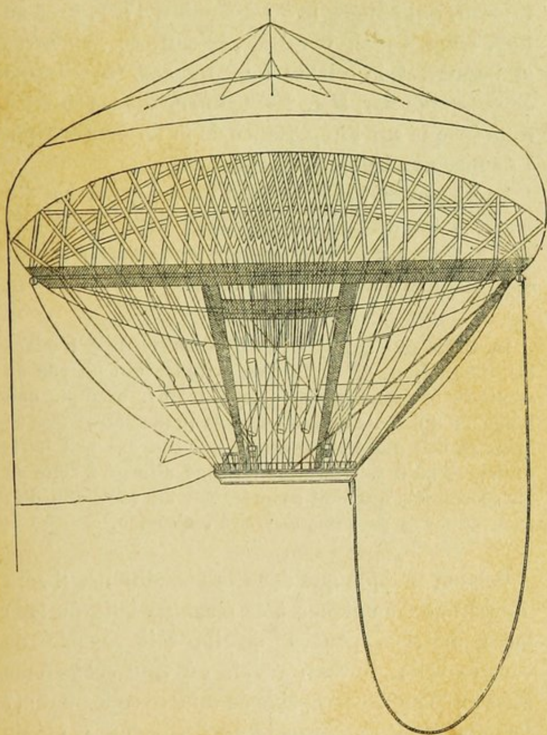
Fig. 45. —_Projet d'aérostat dirigeable du général Meusnier (1784).
