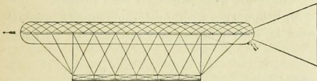
Fig. 70. — Aérostat propulsif de Gontier-Grisy (1862).
