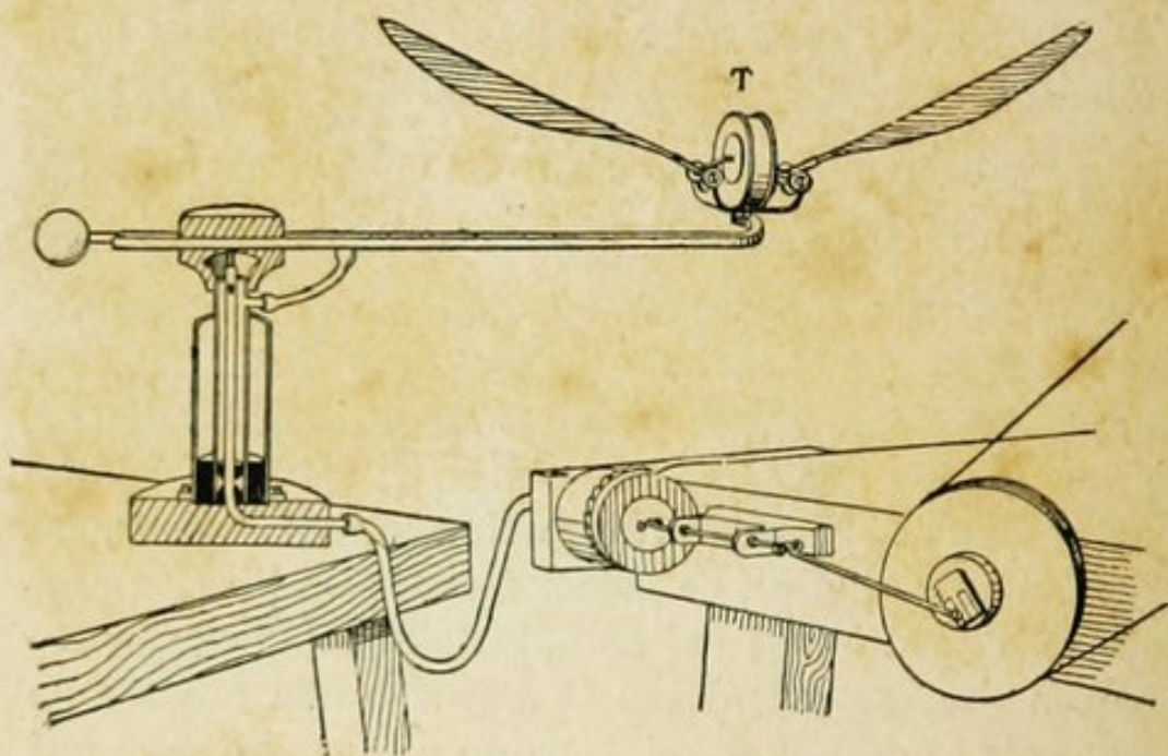
Fig. 12. — Insecte mécanique de M. Marey.
