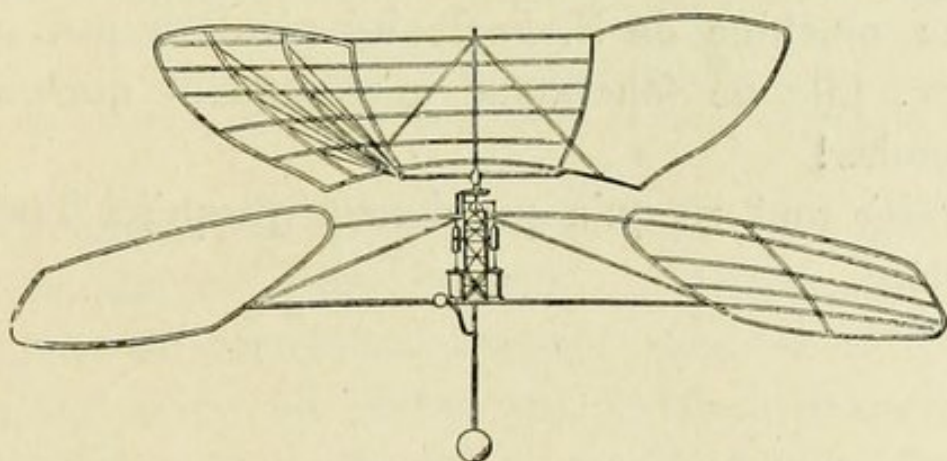
Fig. 50. — Hélicoptère à vapeur de M. Forlanini (1878).
