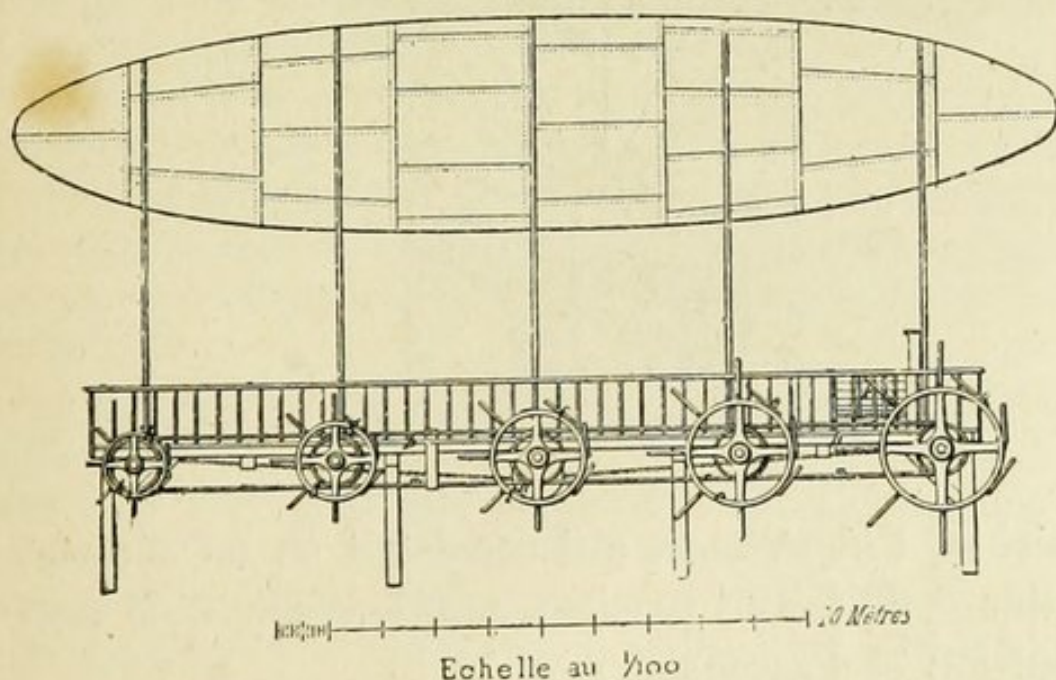
Fig. 71. — Projet d'un ballon de cuivre par Chéradame (1865).
