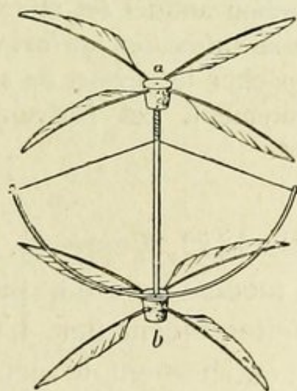
Fig. 25. — Hélicoptère de sir Georges Cayley (1793).
