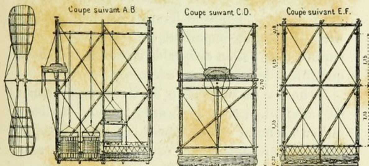
Fig. 90. — Nacelle de l'aérostât électrique de MM. Tissandier frères.
