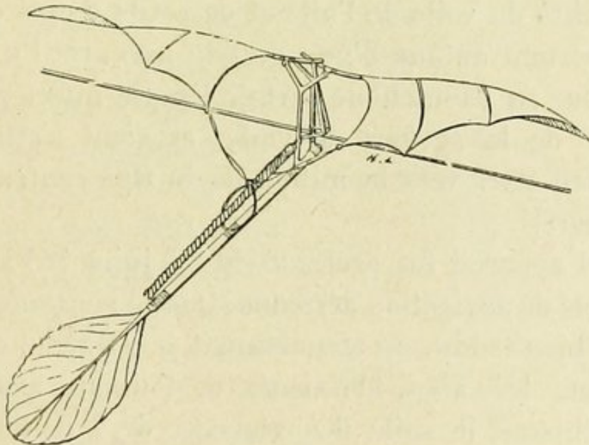
Fig. 20. — Oiseau artificiel d'Alphonse Pénaud (1871).
