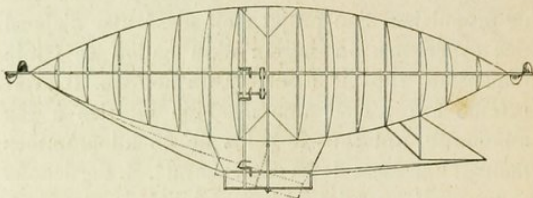
Fig. 76. — Projet d'aérostat en aluminium de Micciollo-Picasse (1871).
