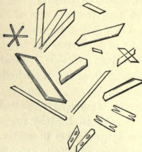
Fig. 2.—INOSITE.
