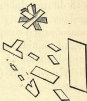
Fig. 1.—MILK-SUGAR.
