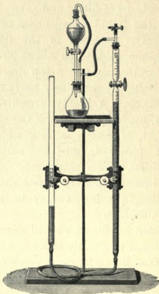
Fig. 7.—NITROGEN-EVOLUTION APPARATUS.
