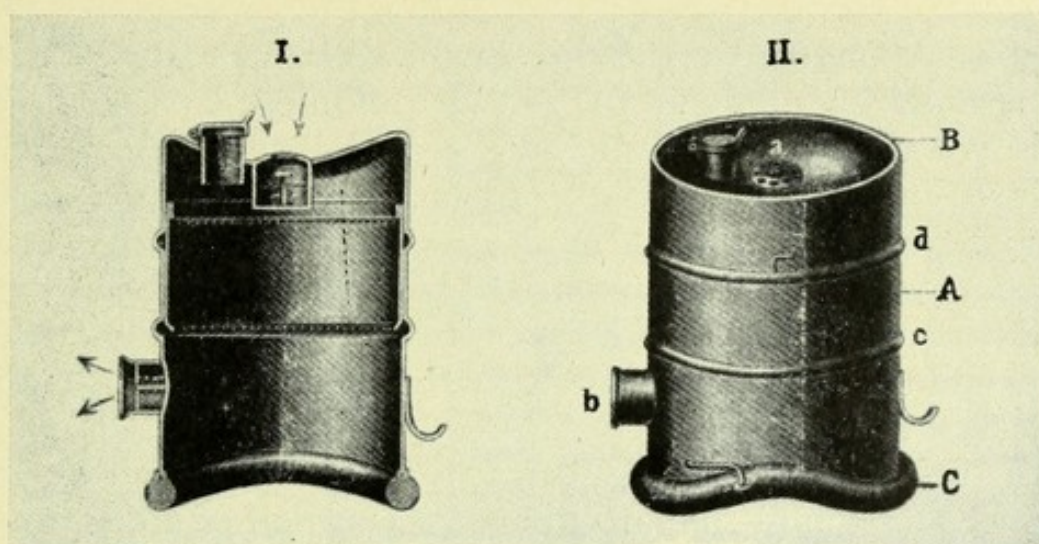
FIG. 156.—WAGNER-LONGARD ETHER INHALER
