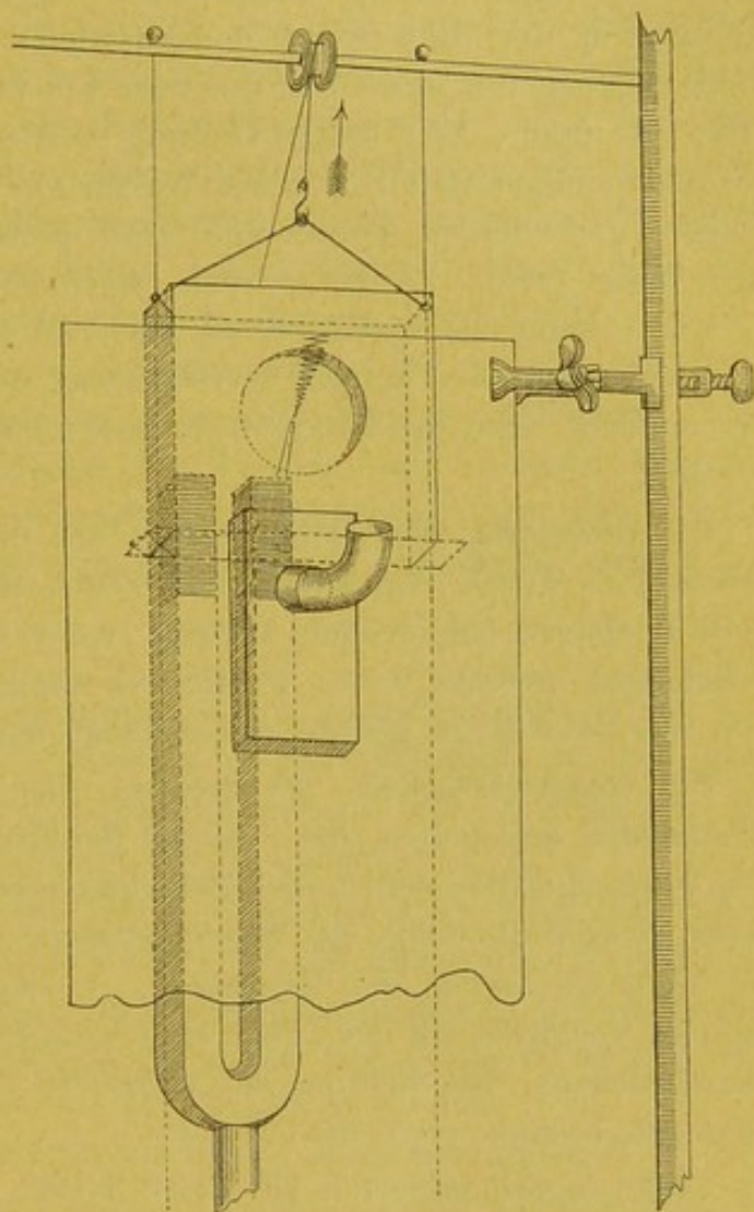
Ermittlung der kürzesten Expositionsdauer eines Riechstoffs, welche zur Hervorbringung einer Geruchsempfindung genügt.
