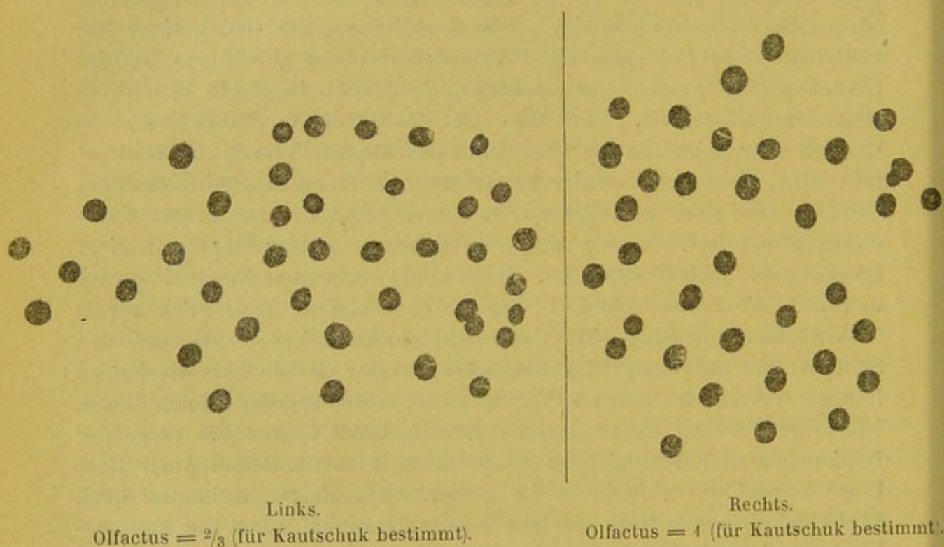
Fig. 40. Riechfelder.
