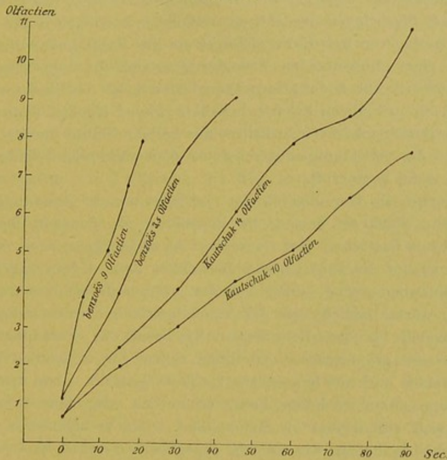
Ermüdungskurven.
