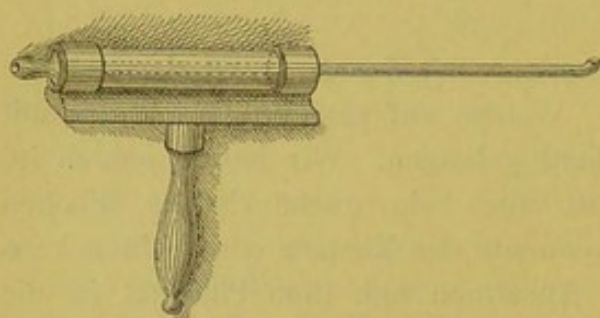
Gustatorischer Riechmesser,
