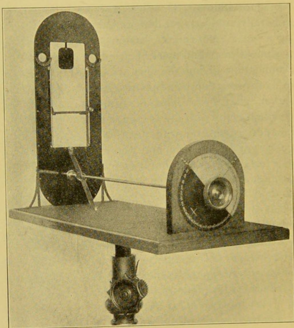
FIG. 15.—JENNINGS' SKIASCOPIC DISC.
