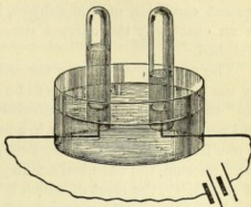
FIG. 8.—VOLTAMETER.
