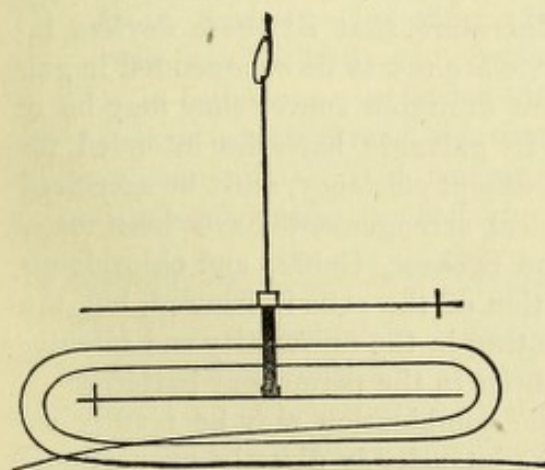
FIG. 9.—GALVANOMETER.
