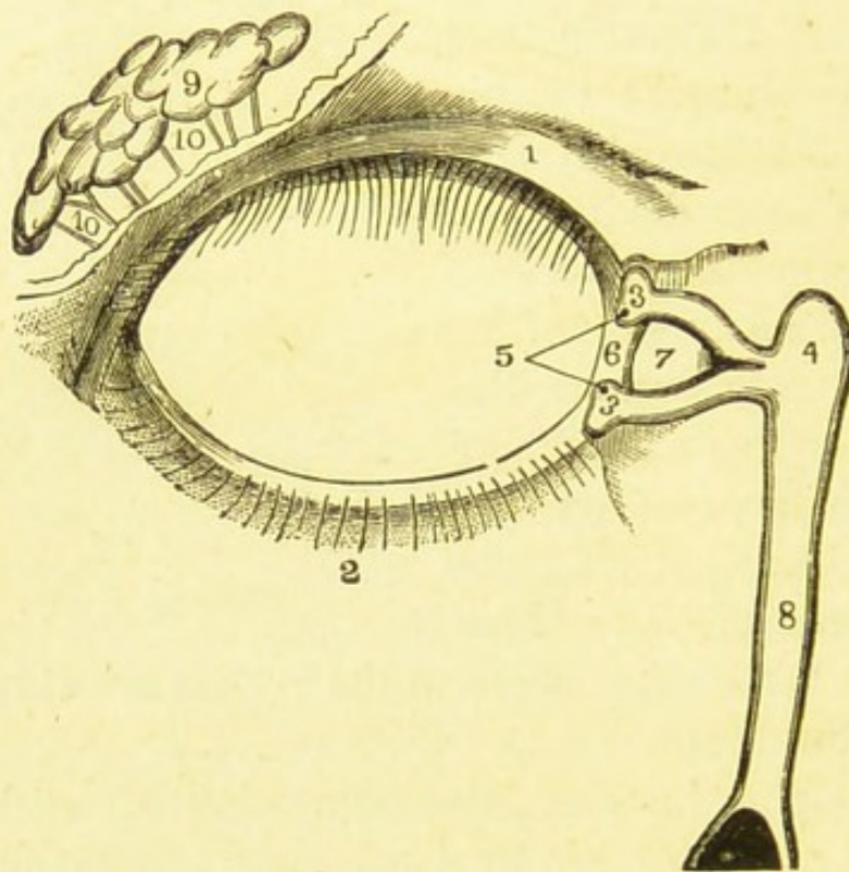
Fig. IV. — Lachrymal Apparatus.
