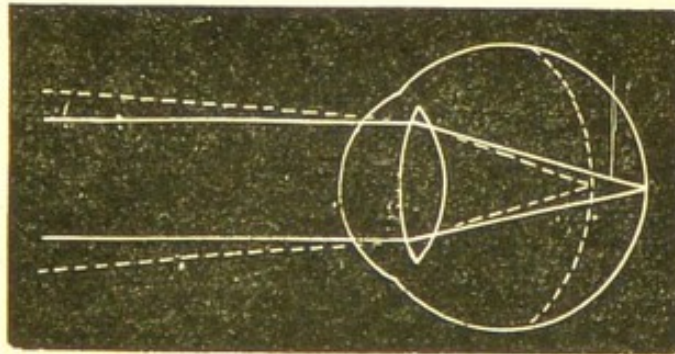
Fig. XVI.—Hypermetropia.
