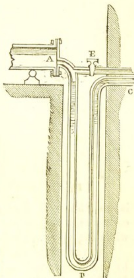
Fig. 60. Siphon.
