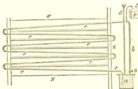
Fig. 65. Bonnemain's Arrangement.
