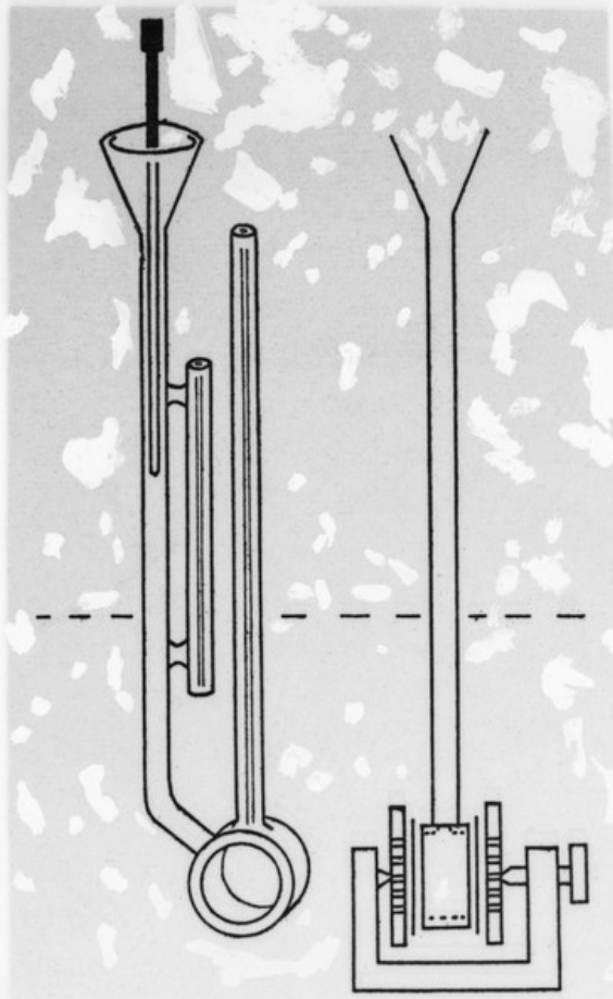
FIG. 2. Zimm-Myerson Osmometer
