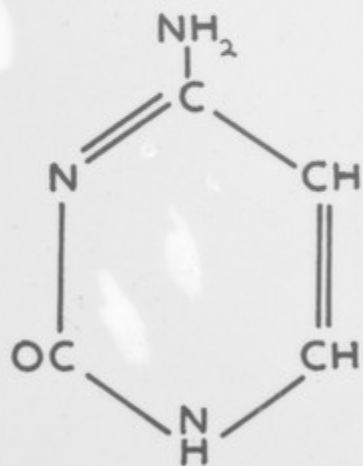
CYTOSINE
