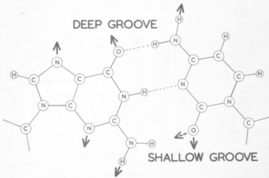
CYTOSINE
