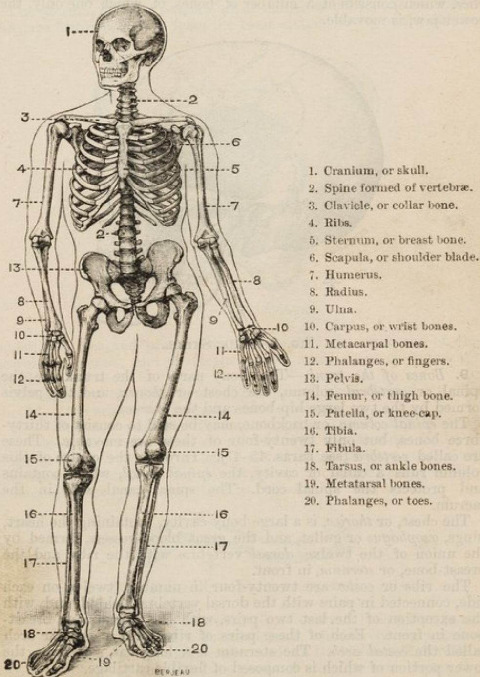
FIG. 1.—THE SKELETON.
