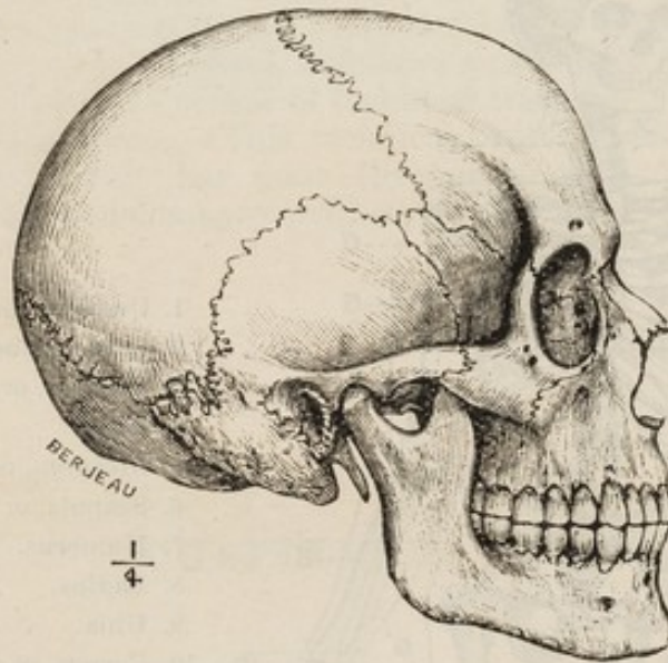
FIG. 2.—THE SKULL.
