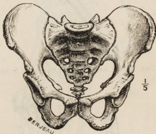
FIG. 3.—THE PELVIS.
