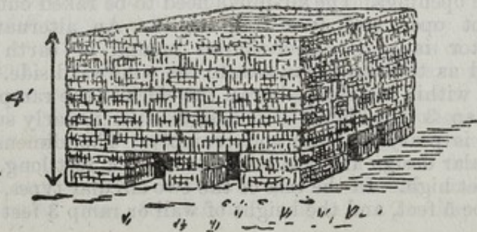
FIG. 18.—CAMP INCINERATOR—RECTANGULAR.
