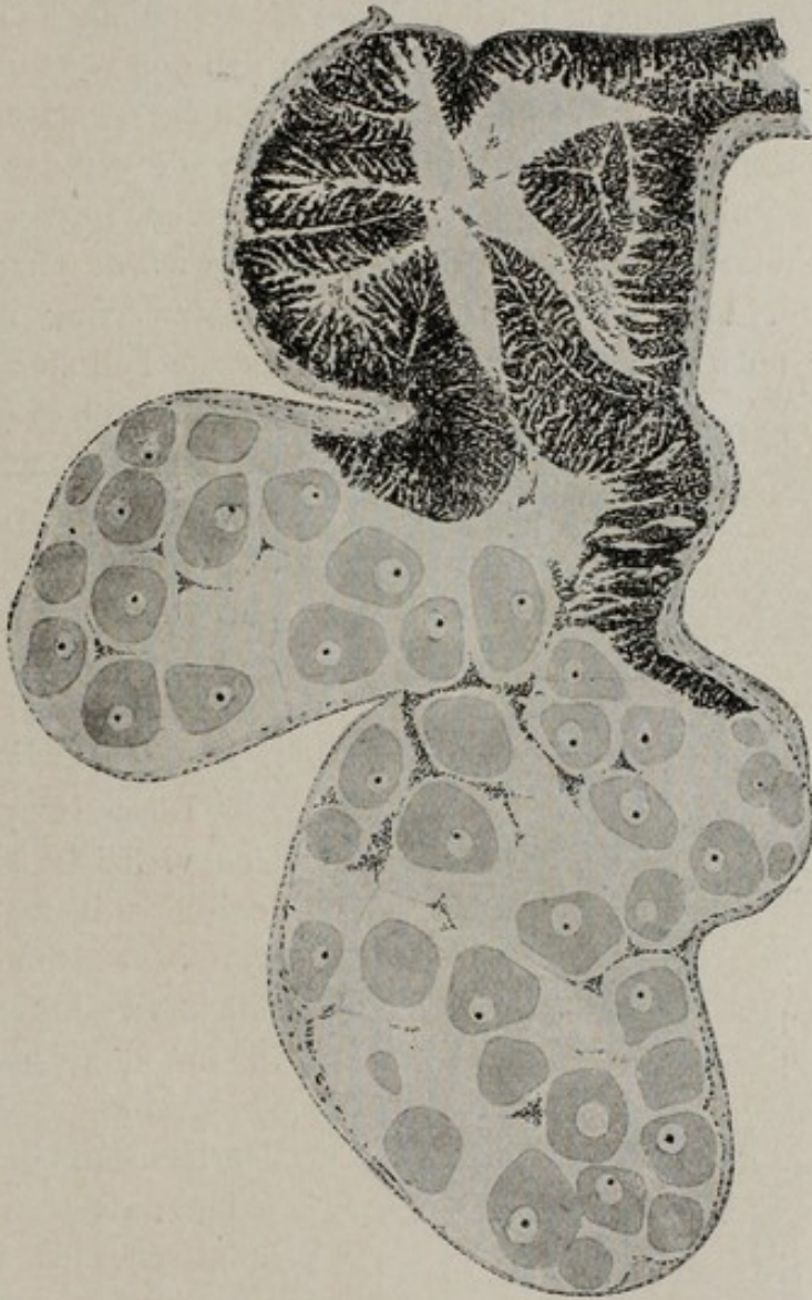
Fig. 89. Schnitt durch den Eierstock eines Seesterns mit eingesprengtem Hodengewebe. Nach Buchner
