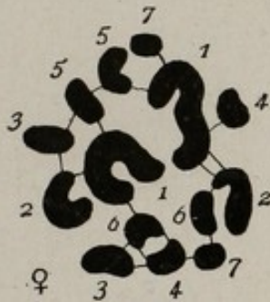
Fig. 24. Chromosomenbestand einer Wanze Jede Sorte ist zweimal vertreten. Nach Wilson
