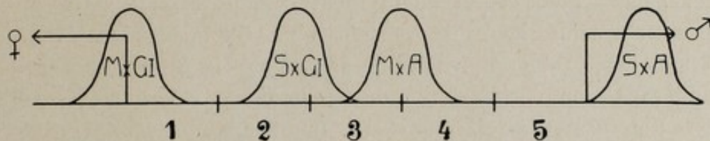
Fig. 49. Intersexualitätsgleichung. Erklärung im Text
