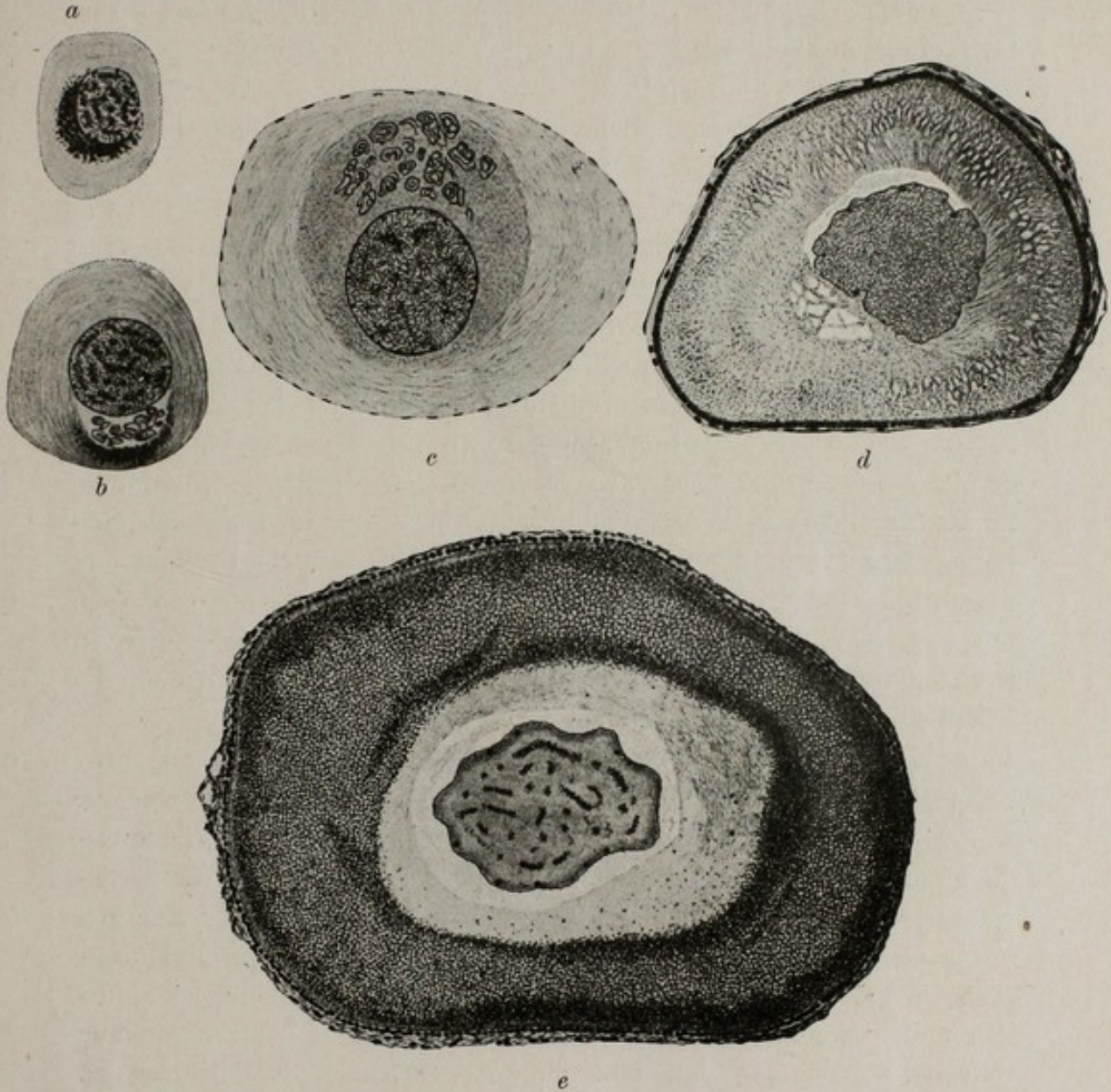
Fig. 5. Fünf Stadien der Ovogenese von Proteus zur Demonstration der Umwandlungen in Plasma und Kern
