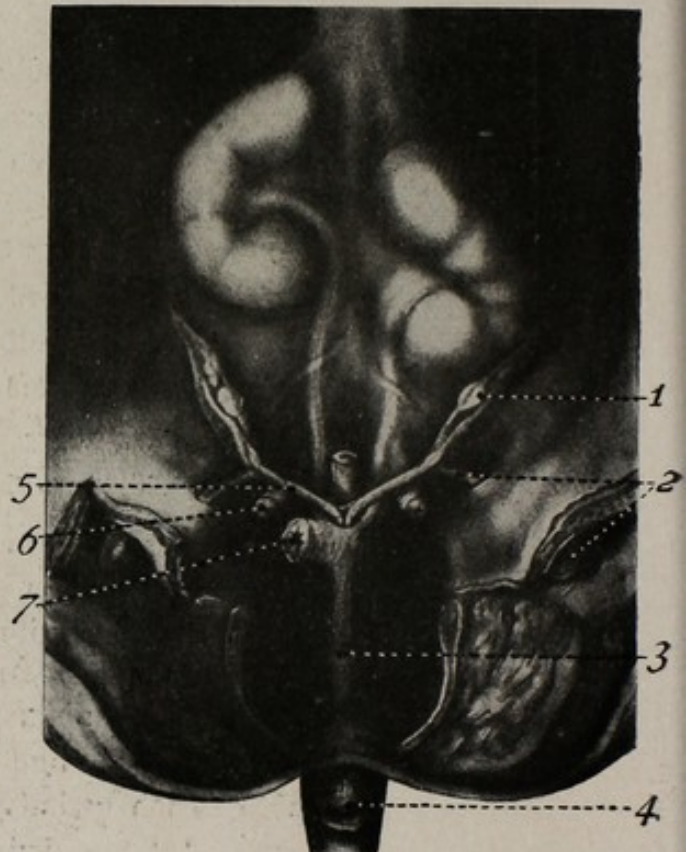
Fig. 59b. Urogenitalapparat einer foetalen Zwicke von 15,5 cm. Gubernaculum und Ausführwege genau wie bei einem Männchen.
