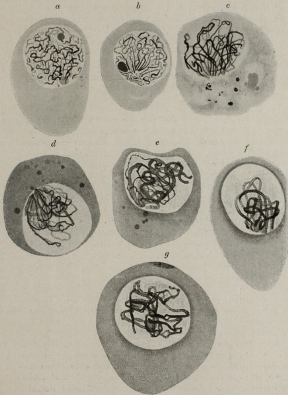
Fig. 20. Die synaptischen Phänomene in der Ovogenese von Dendrocoelum a, b Ausbildung der Chromosomen, c Anordnung zur Parallelkonjugation, d, e die Konjugation, f, g Sichtbarwerden der bivalenten Chromosomen. Nach Gelei
