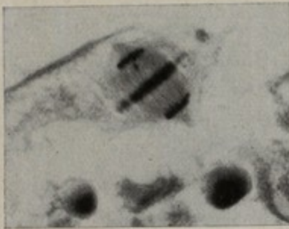
Fig. 36. Reifungsspindeln im Ei von Talaeporia tubulosa . Links das X-Chromosom wandert in den Richtungskörper, rechts das X-Chromosom bleibt im Ei. Mikrophotogramm von Dr. J. Seiler
