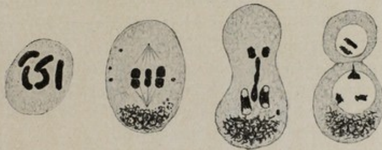
Fig. 38. Reifeteilung bei der Spermatogenese einer Aphide mit Bildung einer ♀ bestimmenden Spermatide (groß, 3 Chromosomen) und einer rudimentären ♂ bestimmenden. Nach v. Baehr
