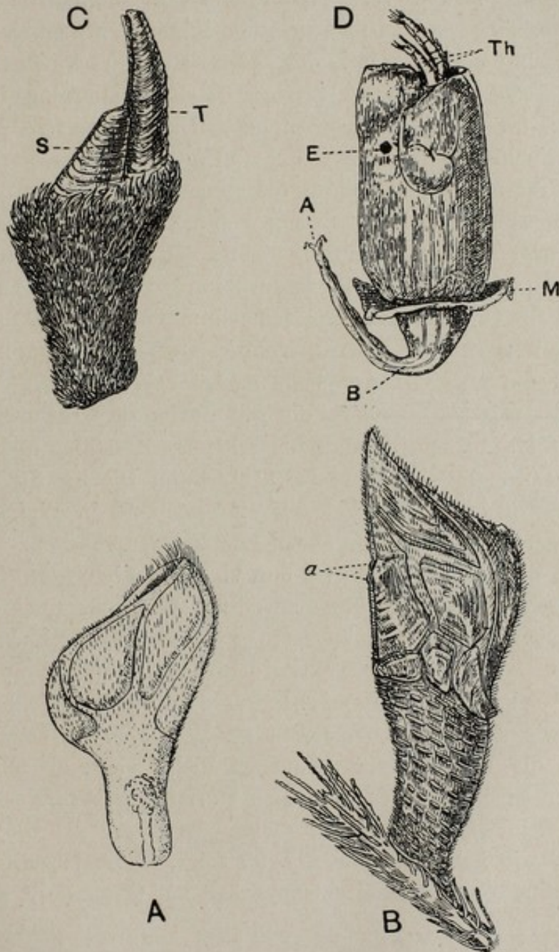
Fig. 98. Geschlechtstiere von Cirrhipedien. Nach G. Smith
