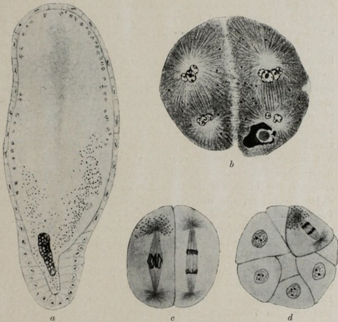
Fig. 4. Typen Keimbahnbestimmender Substanzen
