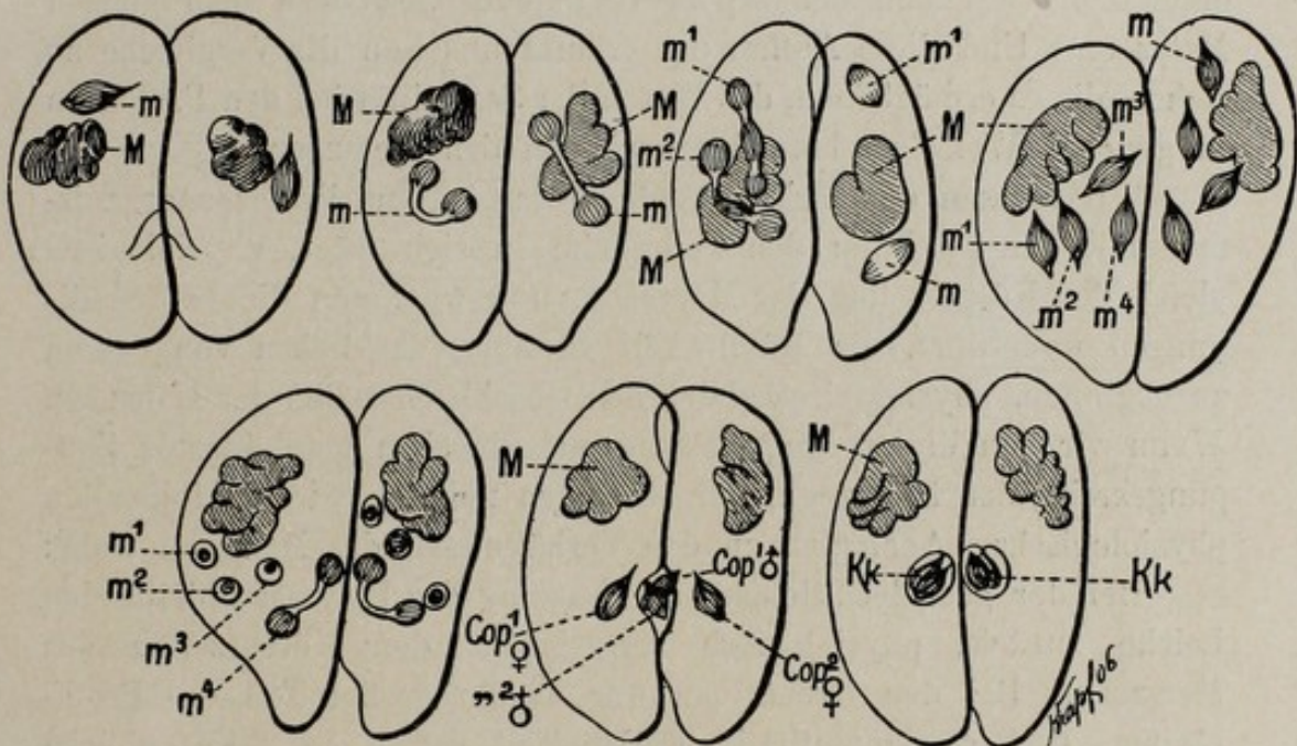
Fig. 11. Schema der Konjugation von Paramecium
