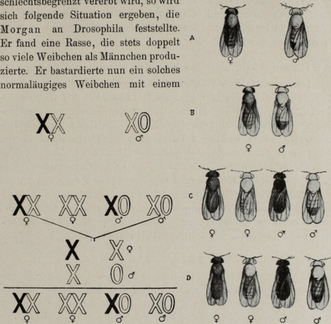
Fig. 105. Schema der Vererbung eines geschlechtsbegrenzten Lethalfaktors bei Drosophila (nach Morgan). Links die Chromosomenverhältnisse; das schwarze X trägt den Lethalfaktor sowie den für rote Augen.
