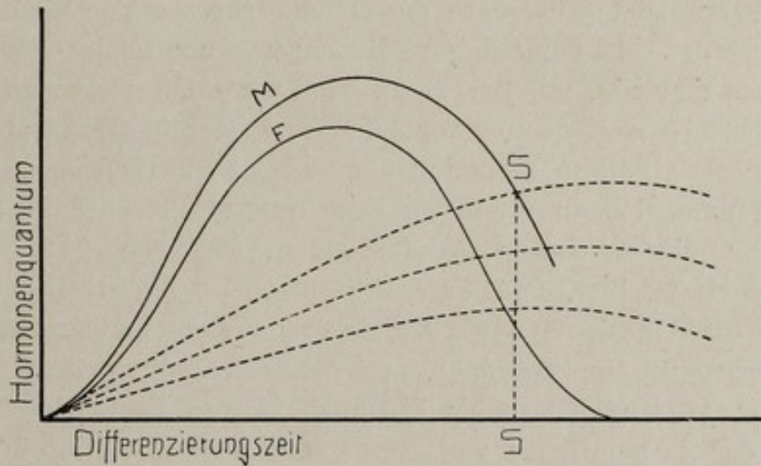
Fig. 73. Kurve zur Interpretation von Hertwigs Froschversuchen.
