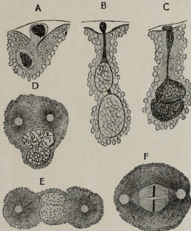
Fig. 101. 6 Stadien der Richtungskörperbildung und Konjugation des Richtungskerns mit dem Eikern bei der parthenogenetischen Artemia .
