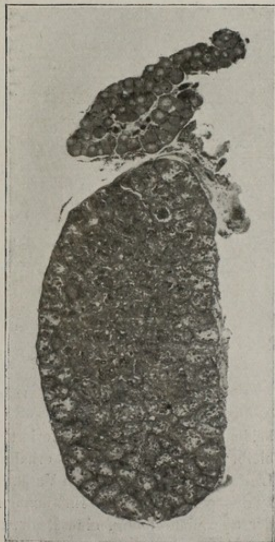
Fig. 85. Biddersches Organ. a. Gesamtansicht der auf den Nieren liegenden Hoden, davor das Biddersche Organ (B. O.), E Müllerscher Gang, U Wolffscher Gang, N Niere, FK Fettkörper Nach Knäppe
