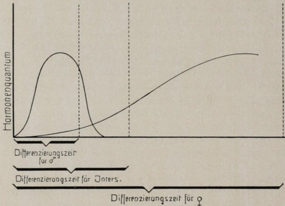
Fig. 65. Kurve zur Interpretation von Baltzers Bonelliaversuchen.
