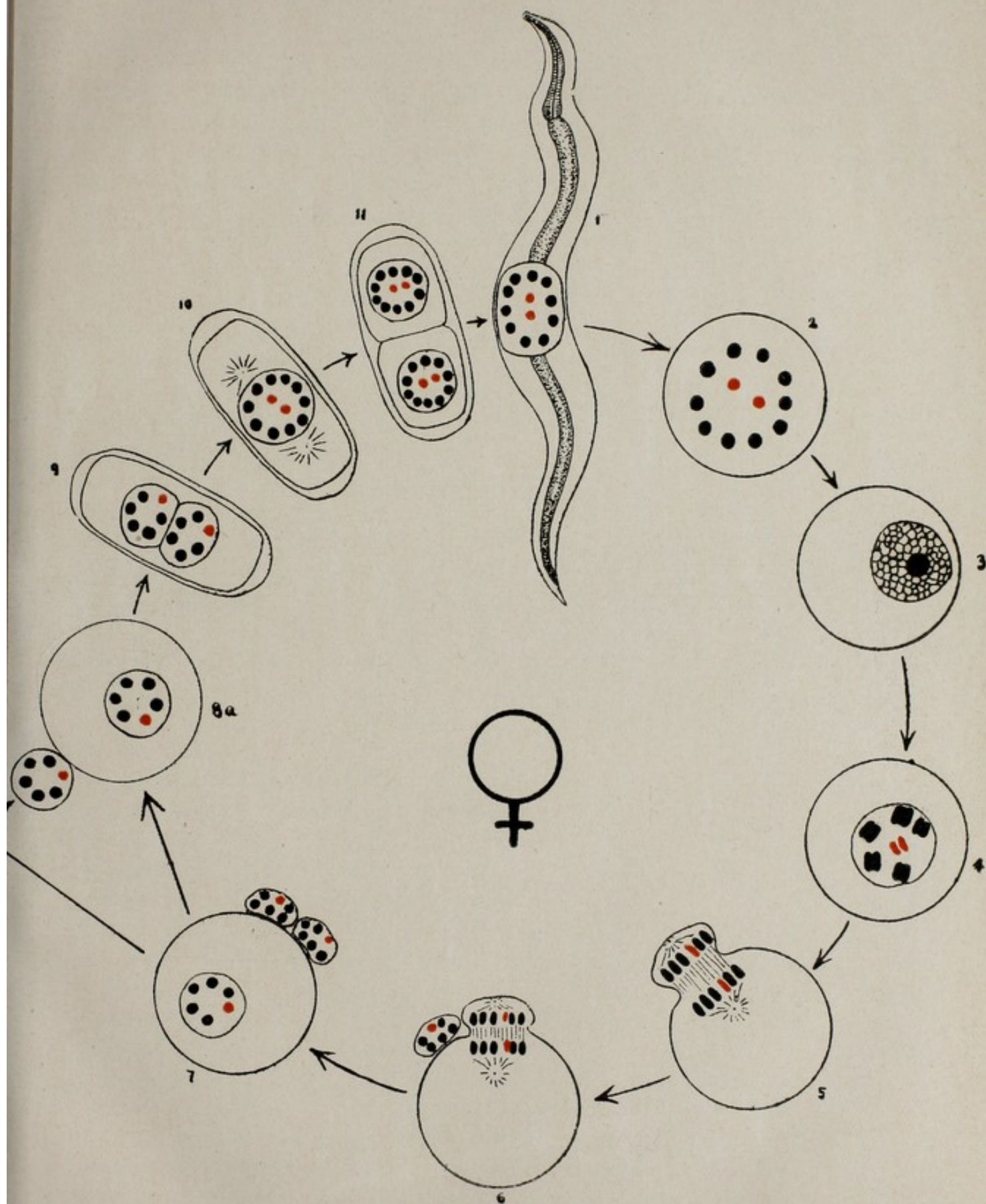
cystidicola. Das X-Chromosom rot. Nach Mulsow
