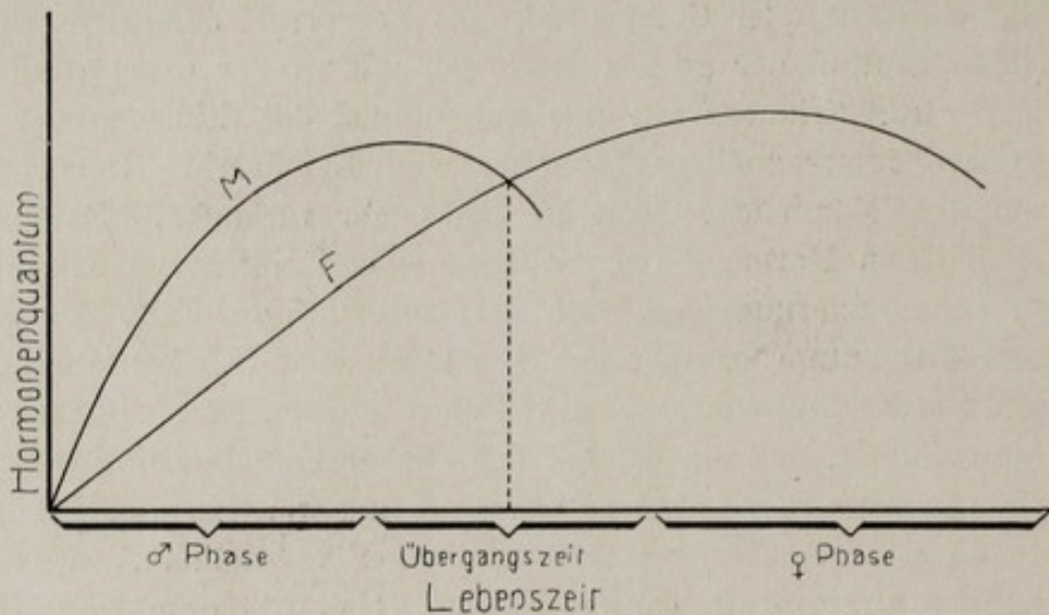
Fig. 97. Kurve zum Geschlechtszyklus der Crepidula
