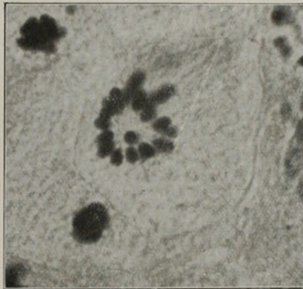
Fig. 25. Photograph des Chromosomenbestandes einer Heuschrecke
