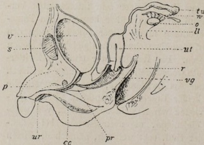
Fig. 112. Drei Typen von ausgesprochenem Pseudohermaphroditismus. Halbschematische Darstellung der Geschlechtsorgane bei Pseudohermaphroditismus.
