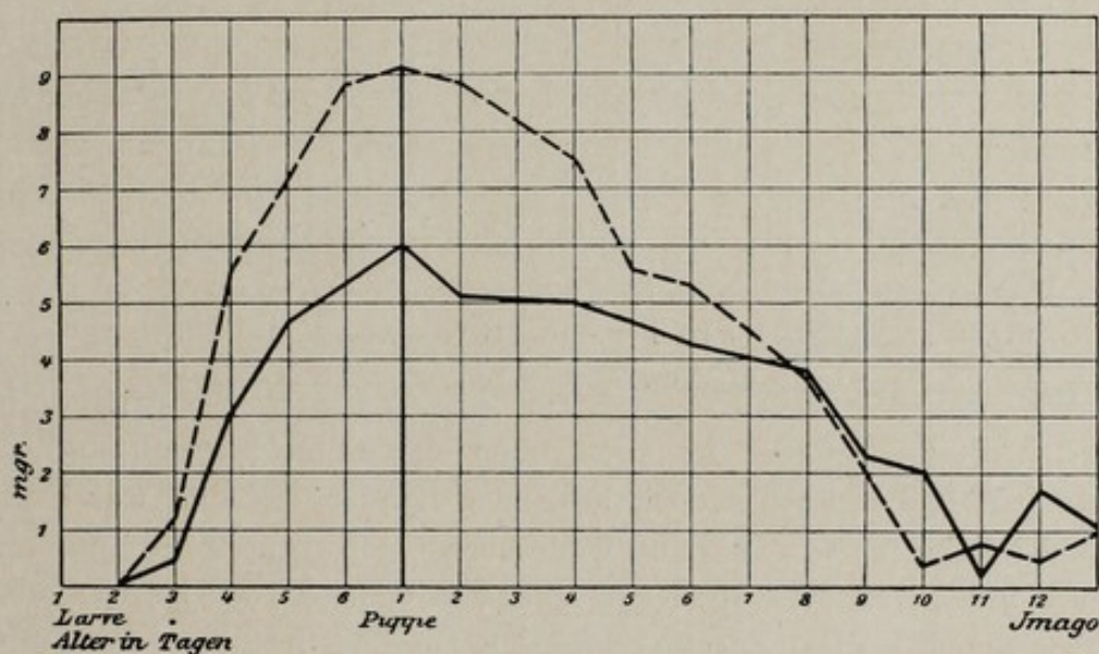
Fig. 61. Änderung im Fett- und Glycogengehalt bei Arbeitsbienen
