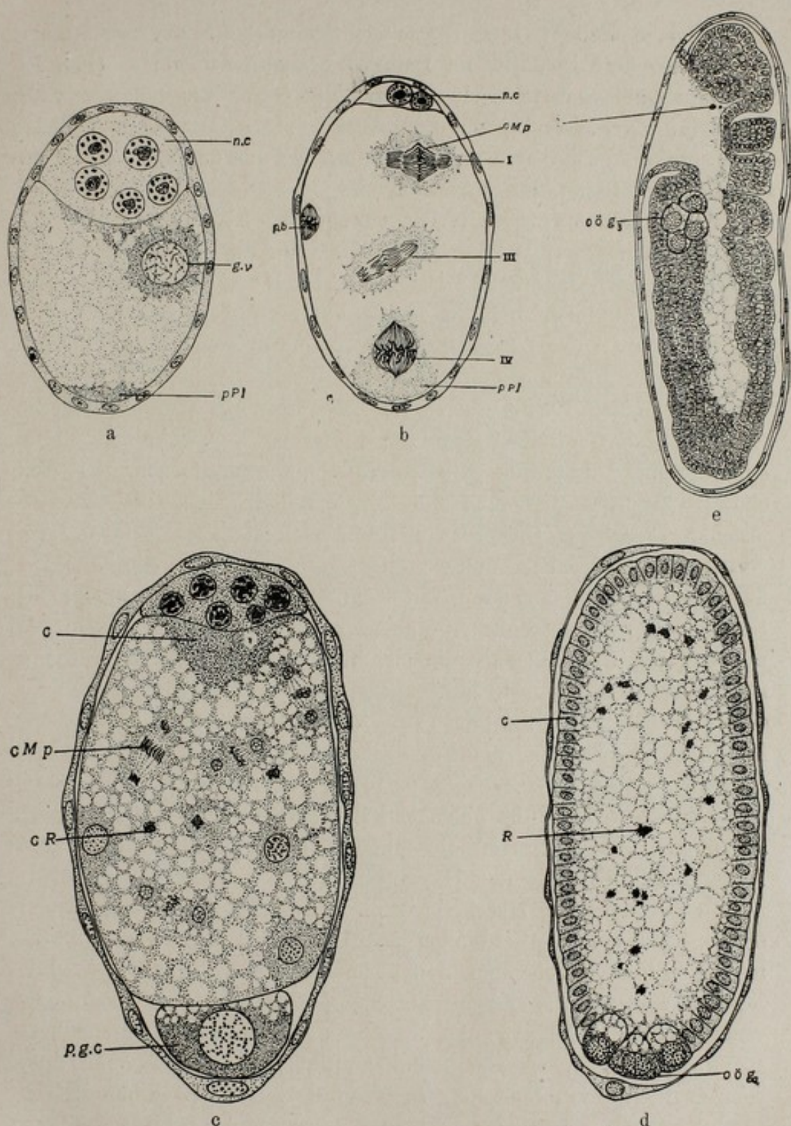
Fig. 3. Die Keimbahn der Gallmücke Miastor
