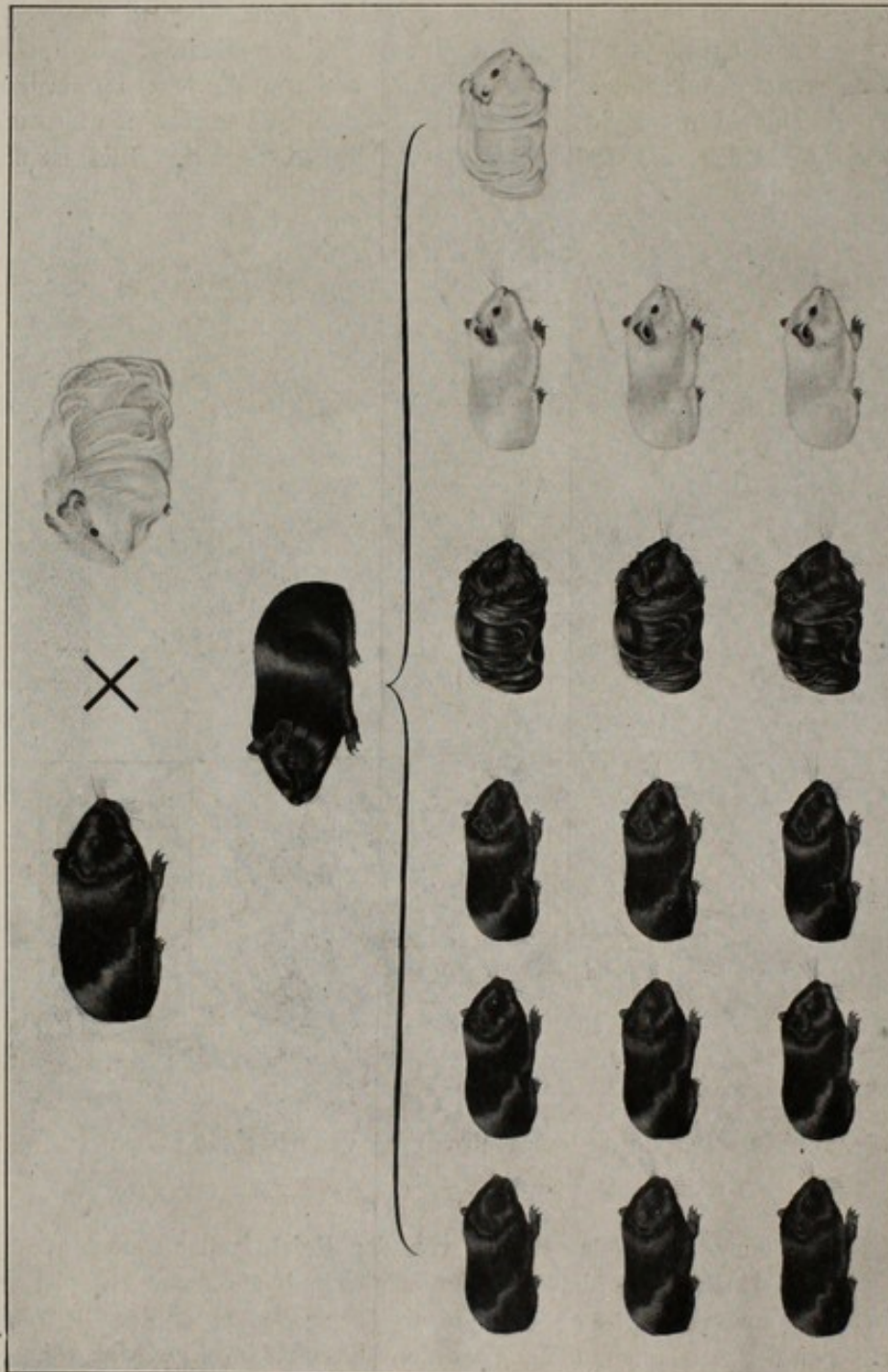
Fig. 14. Dihybride Mendelspaltung bei Kreuzung schwarz-glatthaariger mit weiß-langhaarigen Meerschweinchen. Baur-Goldschmidts Wandtafeln
