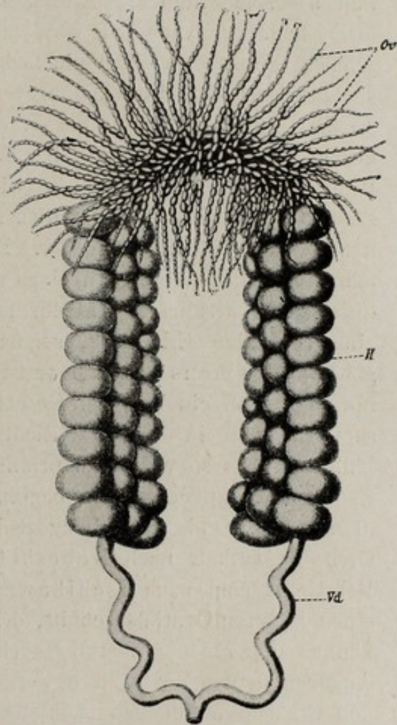
Fig. 86. Geschlechtsapparat von Perla marginata
