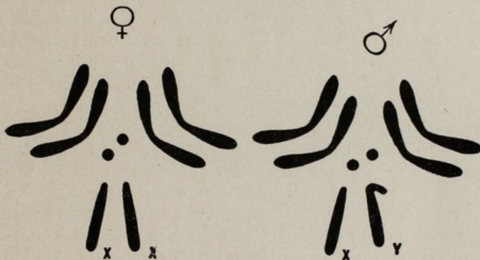
Fig. 40. Chromosomenbestand der weiblichen und männlichen Drosophila , etwas schematisiert. Nach Morgan
