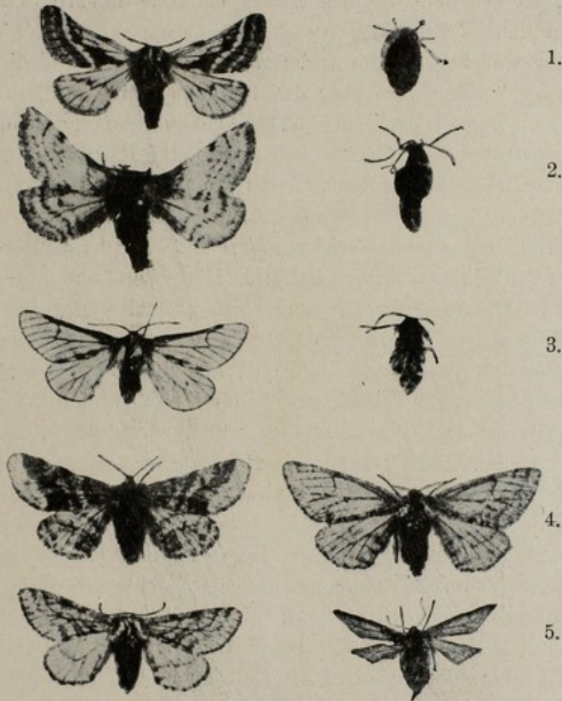
Fig. 52. Bistoniden, links ♂, rechts ♀. 1. Nyssia zonaria. 2. N. graecaria. 3. Poecilopsis rachelae. 4. Lycia hirtaria. 5. pomonaria ♂ × hirtaria ♀ Nach J. W. H. Harrison
