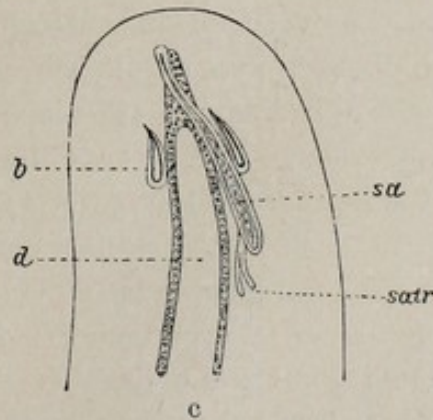
Fig. 64a. Intersexuelle Bonellialarve mit stark weiblichem Einschlag. (Nach 1 Tag vom Rüssel entfernt, dann 10 Tage freie Entwicklung.) — b mittleres Intersex desgl. — c Vorderende eines stark intersexuellen, fast männlichen Individuums.
