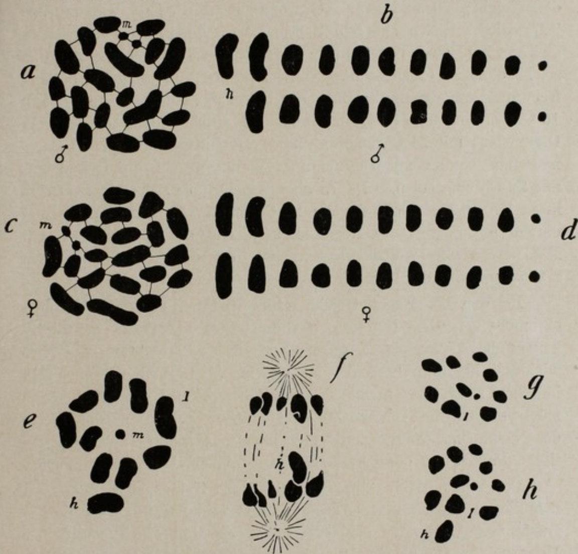
Fig. 31. Chromosomenverhältnisse von Anasa tristis
