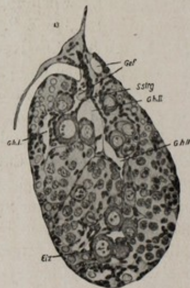
Fig. 68. Rana temporaria . Etwas älterer Eierstock.
