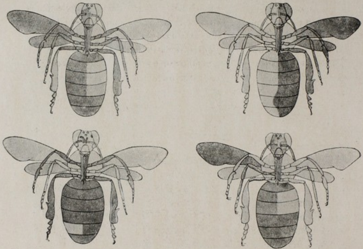
Fig. 80. Schematische Darstellung von vier Euglossinen Bienengynandromorphen Männliche Teile hell, weibliche dunkel. Nach Mehling
