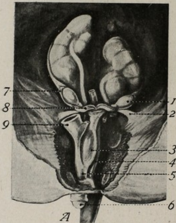
Fig. 59a. Urogenitalapparat eines weiblichen Rinderfoetus von 17 cm
