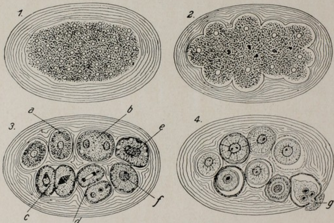
Fig. 10. Fortpflanzung von Aktinosphärium, kombiniert.
