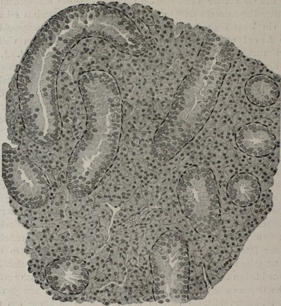
Fig. 53. Schnitt durch einen Säugetierhoden mit Samenkanälchen und interstitieller Drüse. Nach Tandler-Grosz
