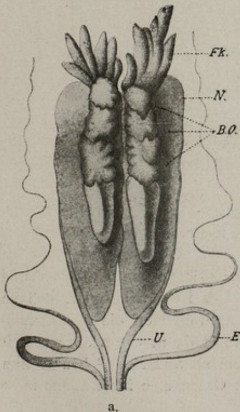
Fig. 85. Biddersches Organ. a. Gesamtansicht der auf den Nieren liegenden Hoden, davor das Biddersche Organ (B. O.), E Müllerscher Gang, U Wolffscher Gang, N Niere, FK Fettkörper Nach Knäppe
