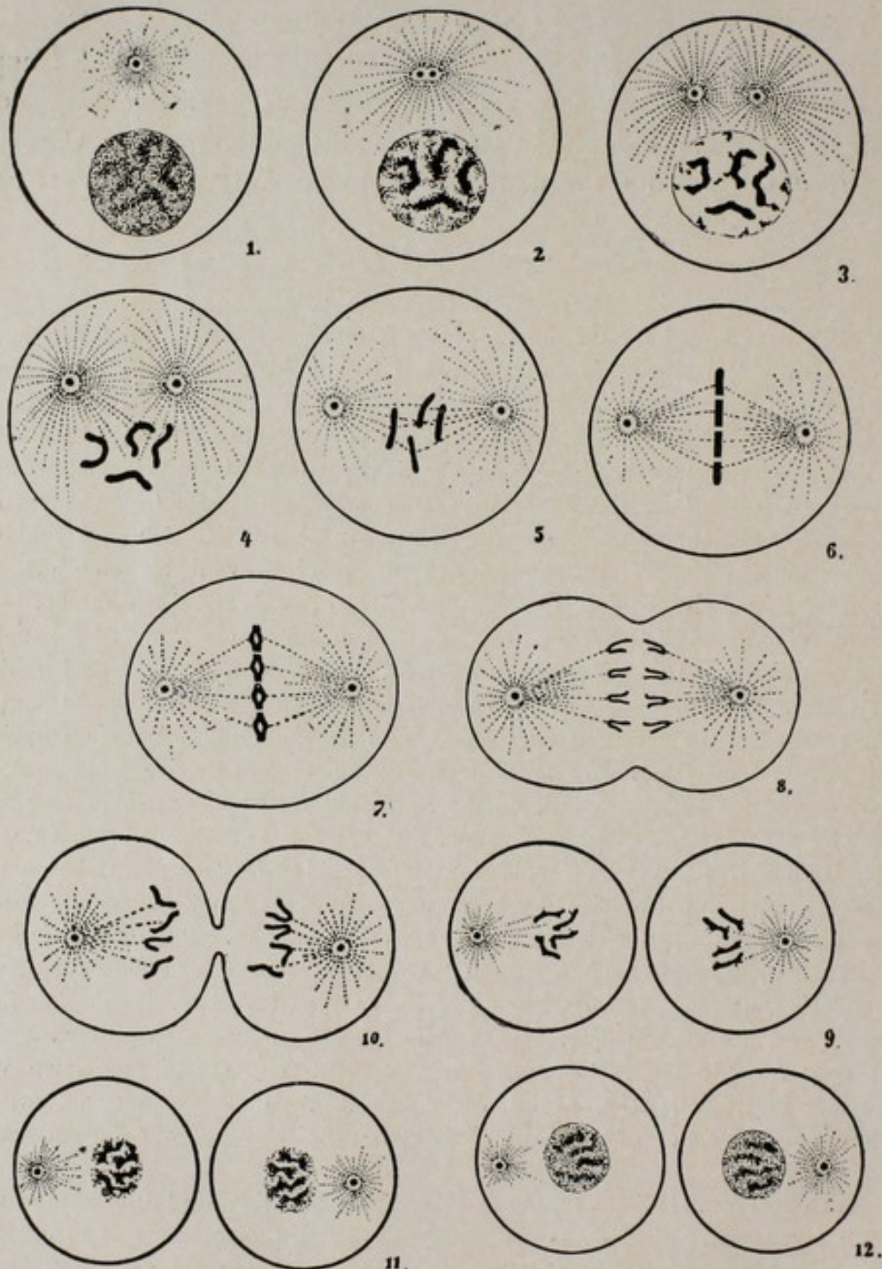
Fig. 18. Schema der mitotischen Zellteilung
