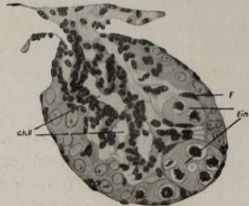
Fig. 67. Rana temporaria . Junger Eierstock.
