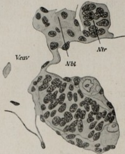
Fig. 66. Junges Bildungsstadium der indifferenten Keimdrüse von Rana temporaria .
