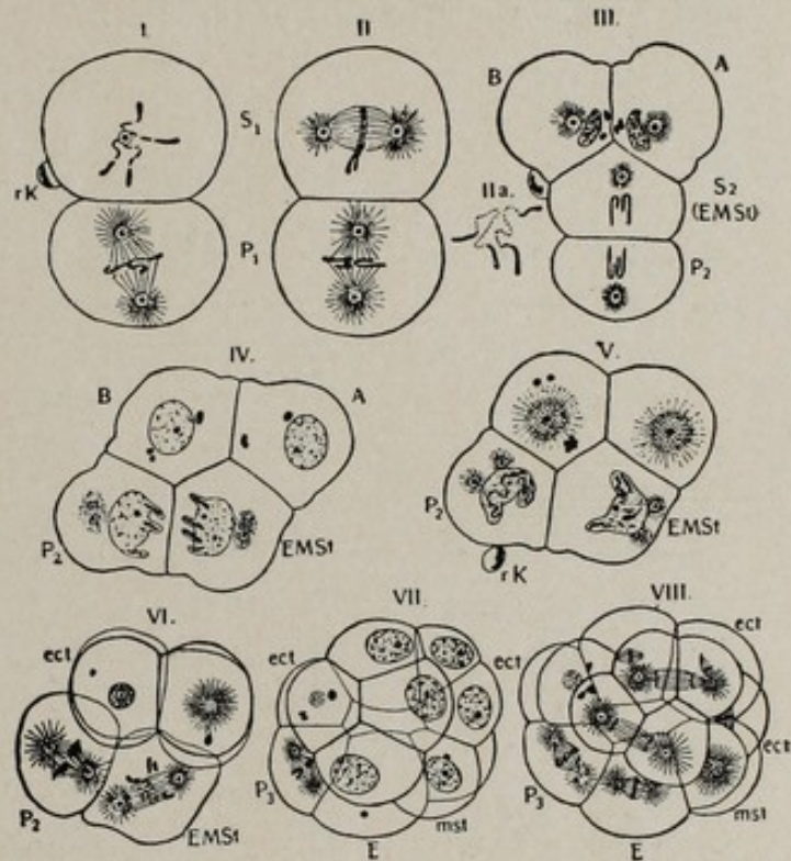
Fig. 1. Acht Furchungsstadien von Ascaris megalocephala zur Demonstration der Chromatindiminution. S_1 die Ursomazelle, P_1 — P_3 die Stammzellen der Geschlechtszellen, S_2 die 2. Ursomazelle (EMSt), E_1 ect Ektodermanlage, mst Anlage von Mesoderm und Stomodäum, rk Richtungskörper, IIa die Chromosomen der Ursomazelle. Nach Boveri aus Harms.
