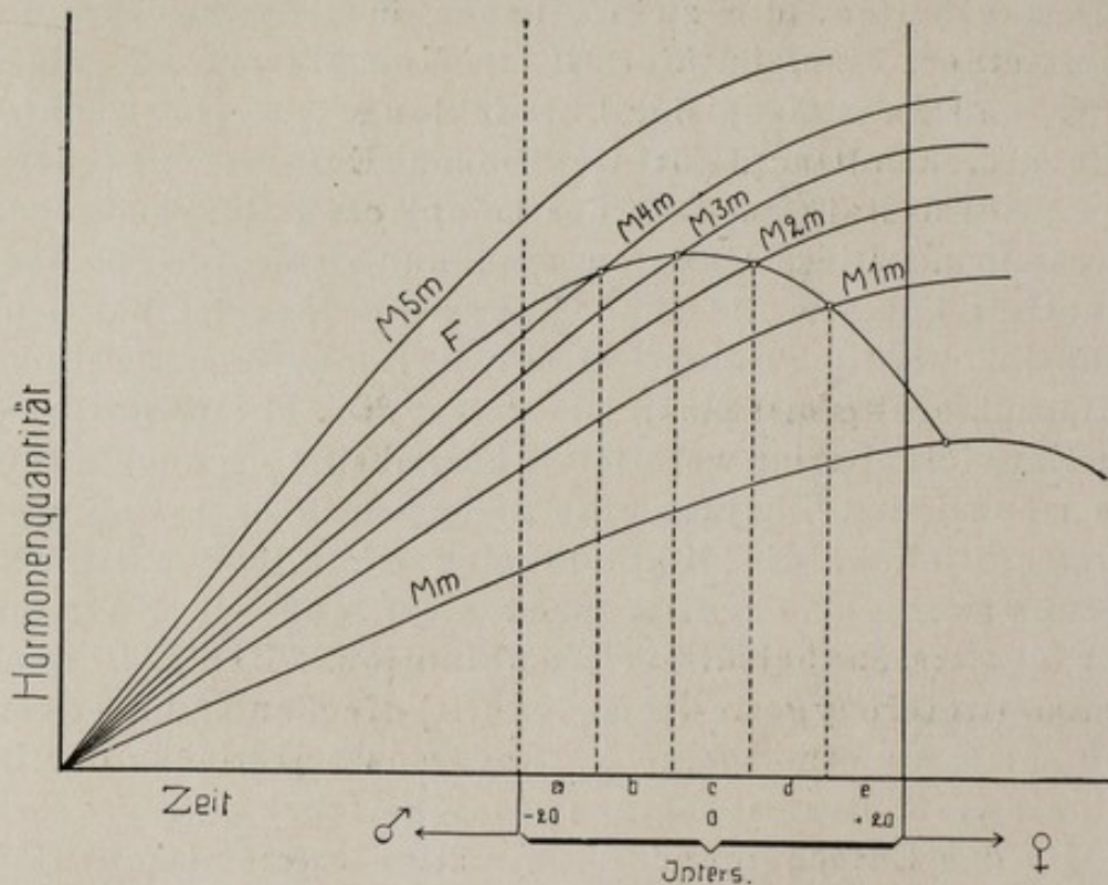
Fig. 51. Kurvenschema zur physiologischen Interpretation der Intersexualität. Erklärung im Text
