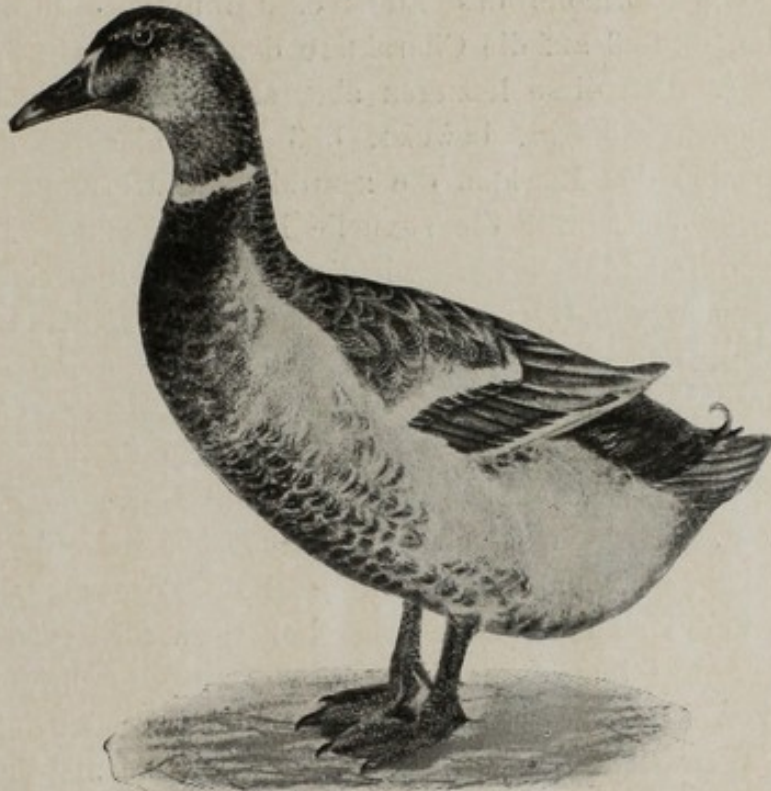
Fig. 55c. Kastrierte Ente. Nach Goodale
