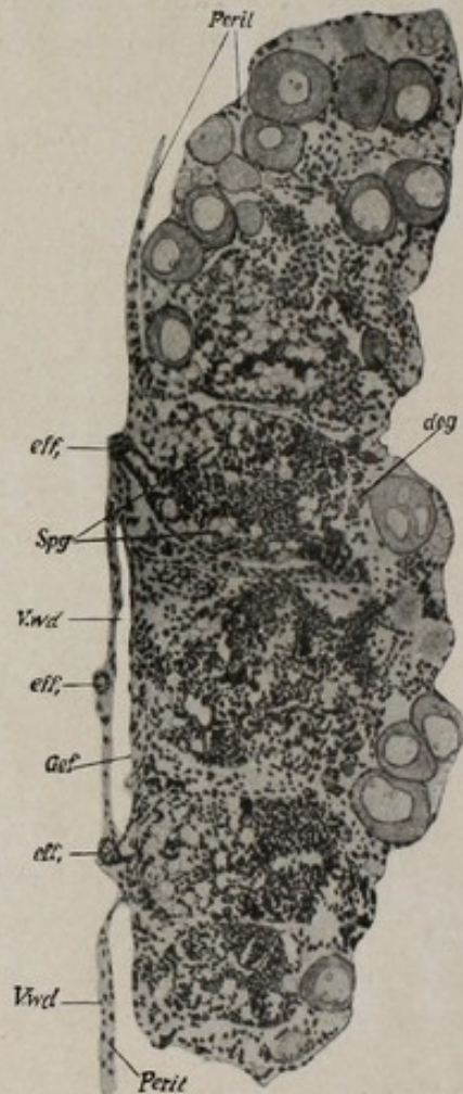
Fig. 72. Keimdrüse eines Fröschchens mit indirekter Hodenentwicklung (Umwandlung)
