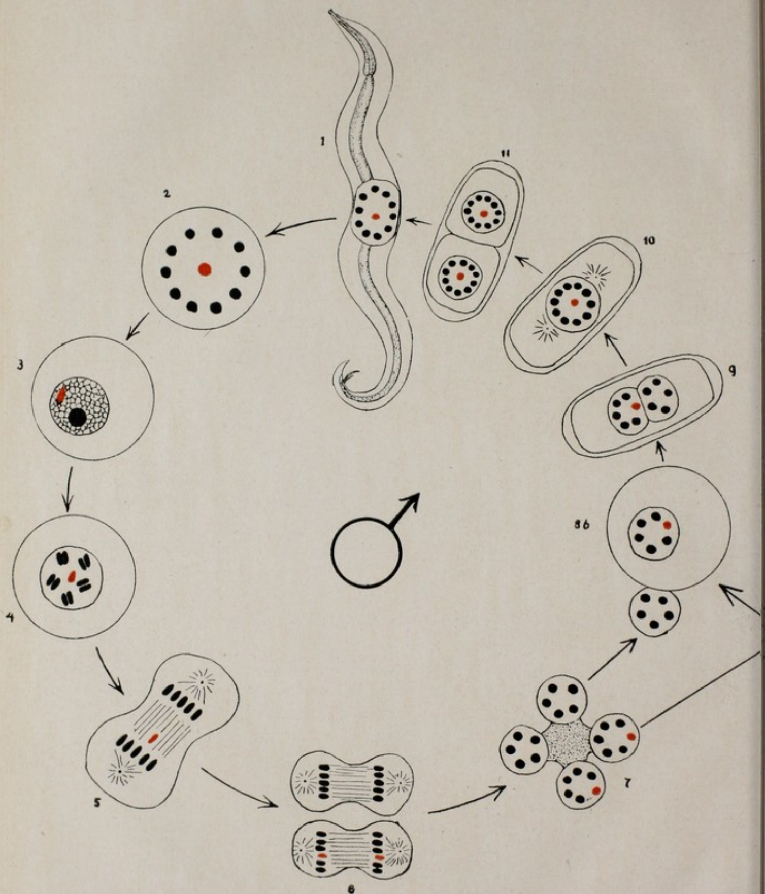
Fig. 32. Schema des Chromosomenzyklus von Ancyra .
