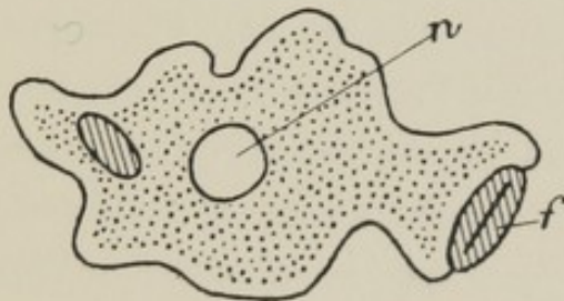
FIG. 17.—AMŒBA.
