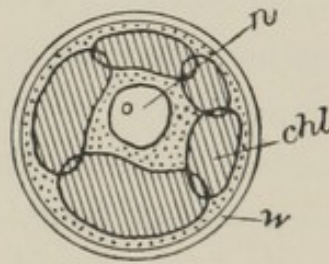
FIG. 18.—PLEUROCOCCLUS.
